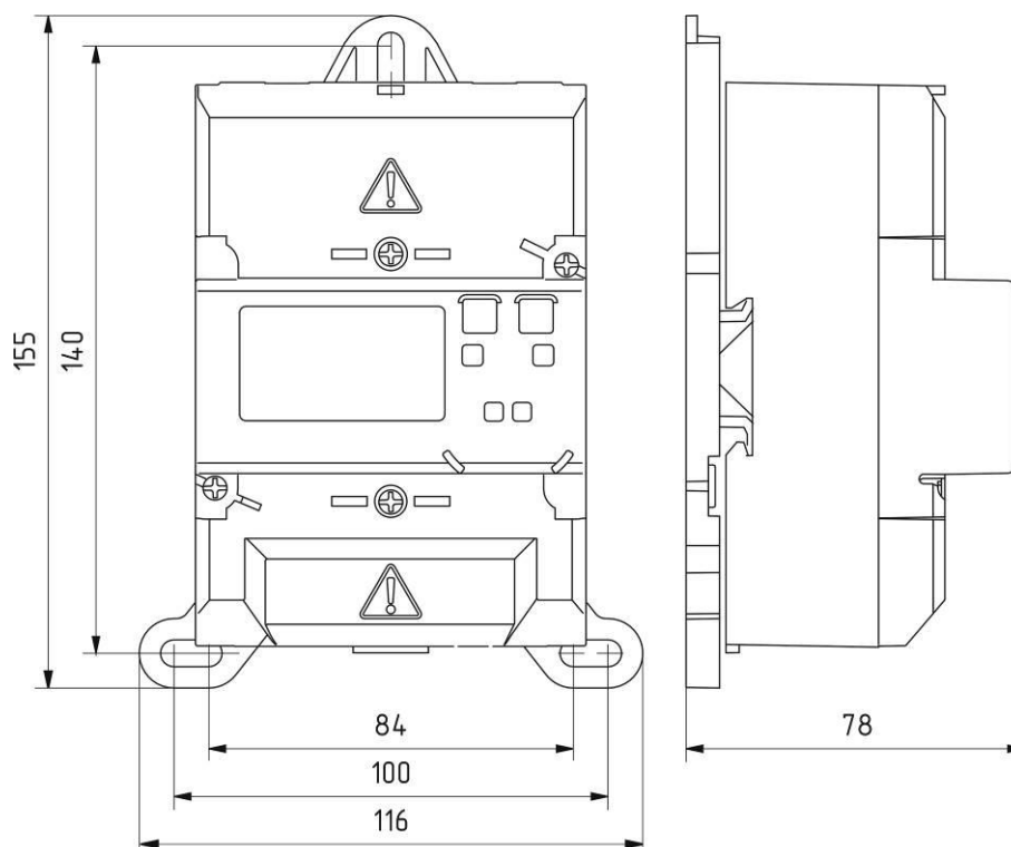
Рисунок В.2 – Тип корпуса D17 с переходной пластиной, позволяющей осуществлять монтаж счетчика на плоскую поверхность с помощью трех винтов
