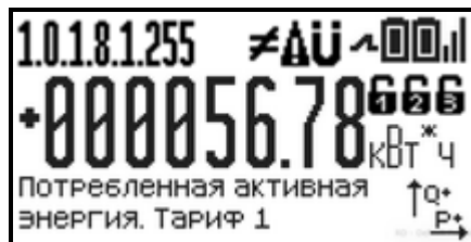
Рисунок 3.3 – Пиктограммы состояния счетчика и электронных пломб
