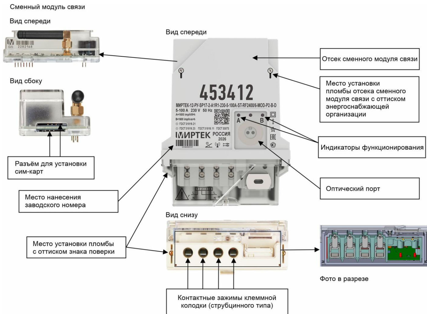
Рисунок Е.2.1 – Тип корпуса SP17 с индикацией и оптическим портом на корпусе
