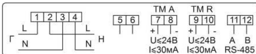
Рисунок Б.22 – Схема включения счетчиков в корпусах W3 с интерфейсом RS-485 и с двумя (независимыми) дискретными выходами, настроенными как телеметрический выход активной энергии (TM A) и реактивной энергии (TM R)
