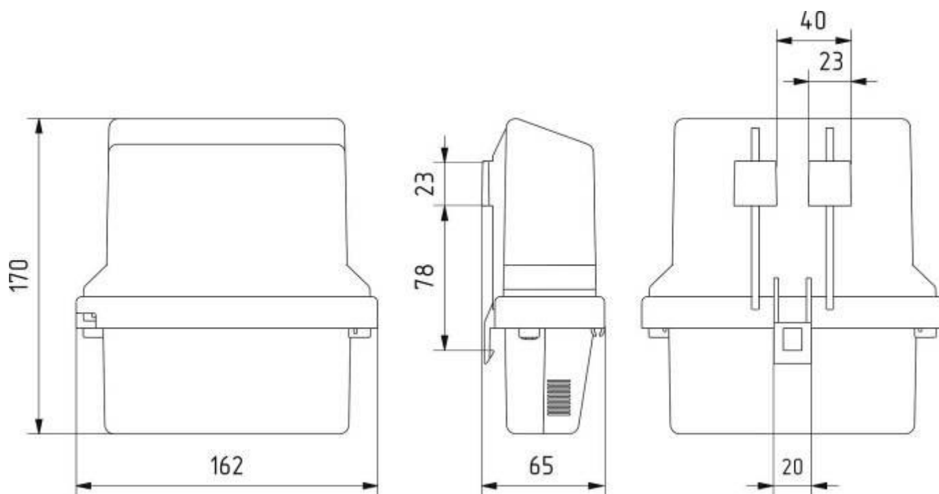
Рисунок В.12 – Тип корпуса SP3
