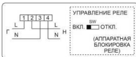
Рисунок Б.33 – Схема включения счетчиков в корпусах W9 и аппаратной блокировкой встроенного реле управления нагрузкой (с помощью микропереключателя)
