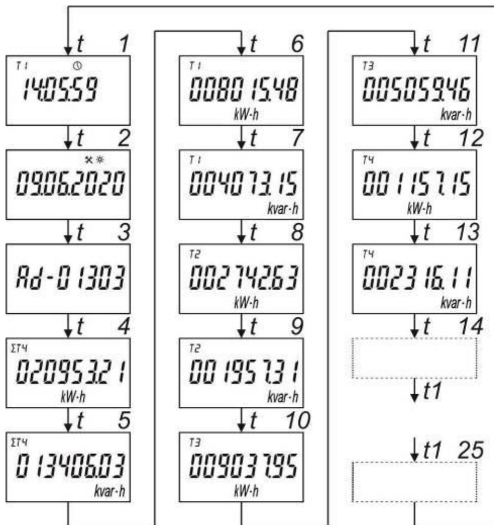
Рисунок 3.10 – Режимы циклической индикации счетчика
