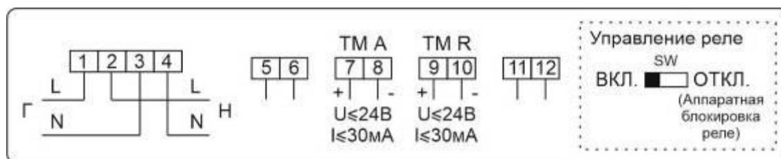
Рисунок Б.24 – Схема включения счетчиков в корпусах W3 с двумя (независимыми) дискретными выходами, настроенными как телеметрический выход активной энергии (ТМ А) и реактивной энергии (ТМ R) и аппаратной блокировкой встроенного реле управления нагрузкой (с помощью микропереключателя)
