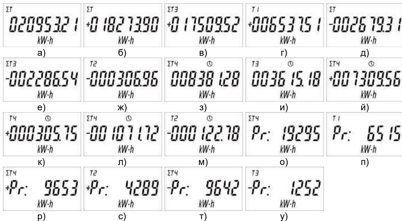
Рисунок 3.11 – Программируемые режимы индикации счетчика
