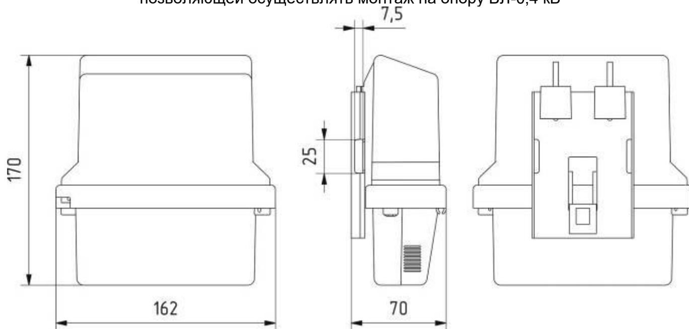
Рисунок В.16 – Тип корпуса SP3 с переходной пластиной, позволяющей осуществлять монтаж на опору ВЛ-0,4 кВ
