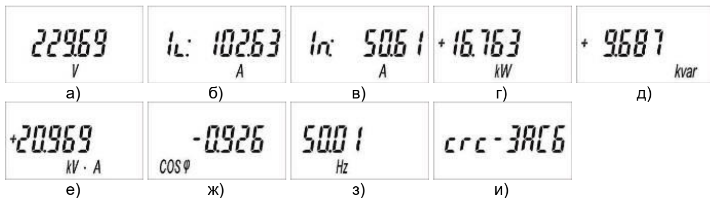
Рисунок 3.13 – Программируемые режимы индикации счетчика
