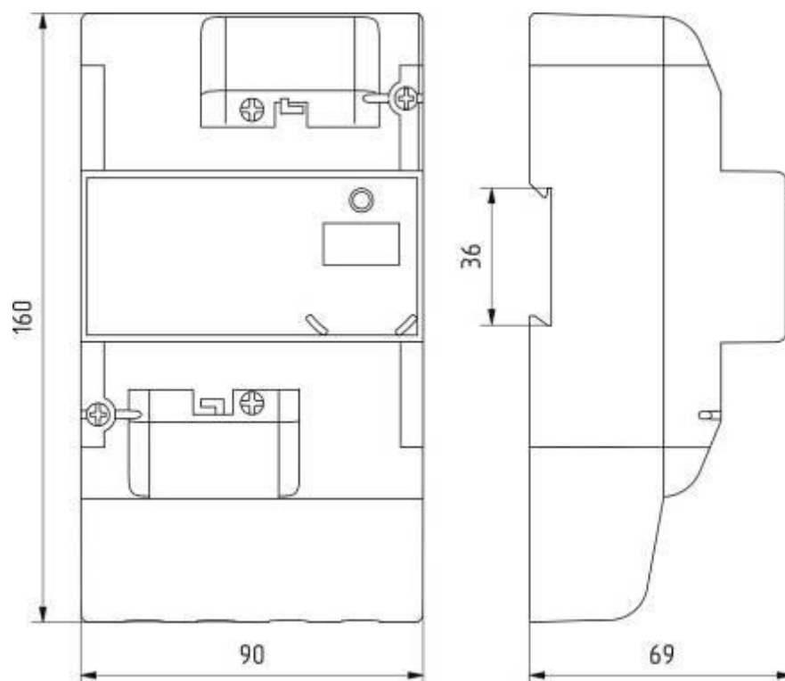
Рисунок В.8 – Тип корпуса D4
