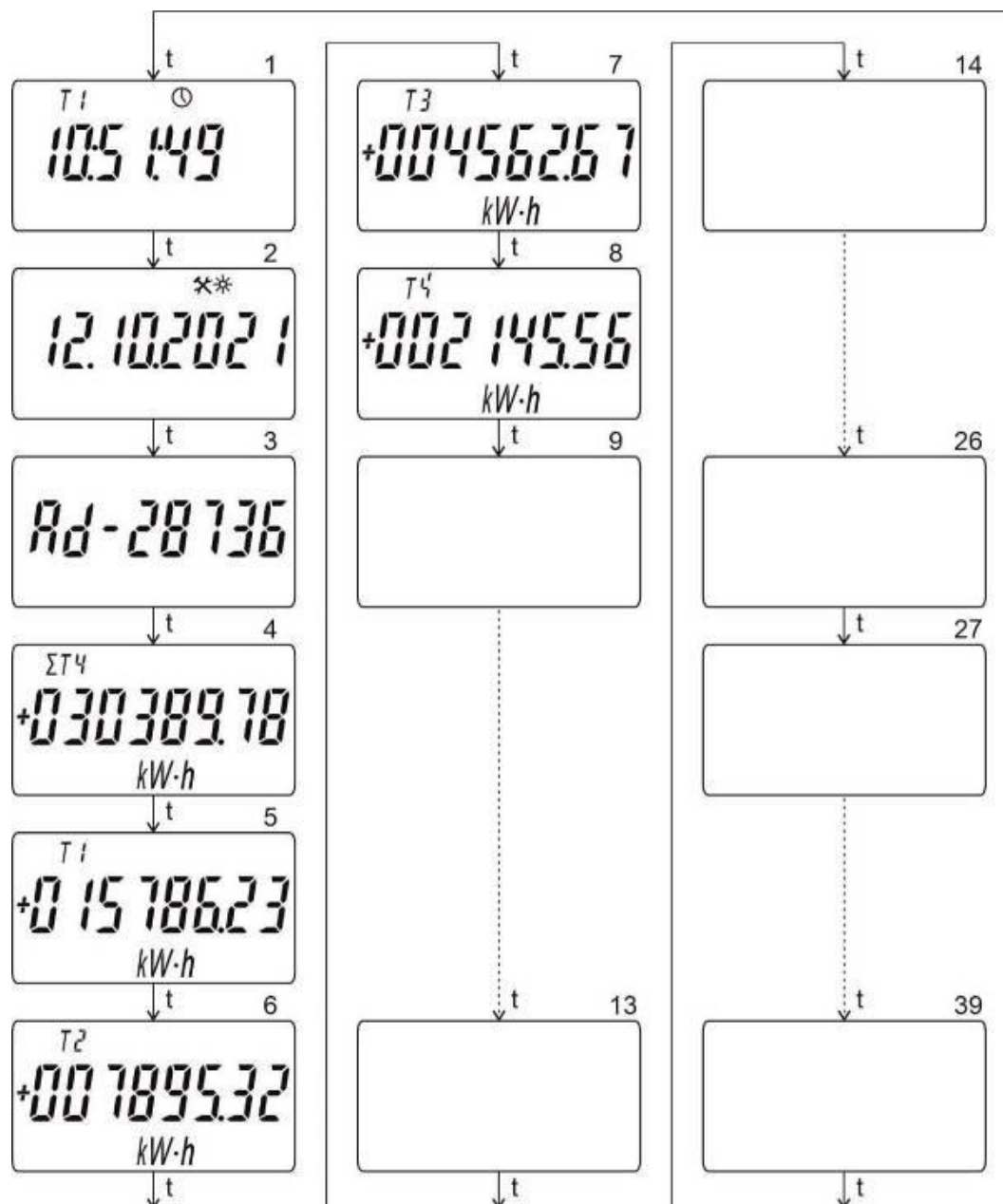
Рисунок 3.14 – Режимы циклической индикации счетчика
