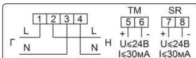
Рисунок Б.13 – Схема включения счетчиков в корпусах W1 с двумя (независимыми) дискретными выходами, один из которых настроен как как телеметрический выход (TM), а второй как реле сигнализации (SR)
