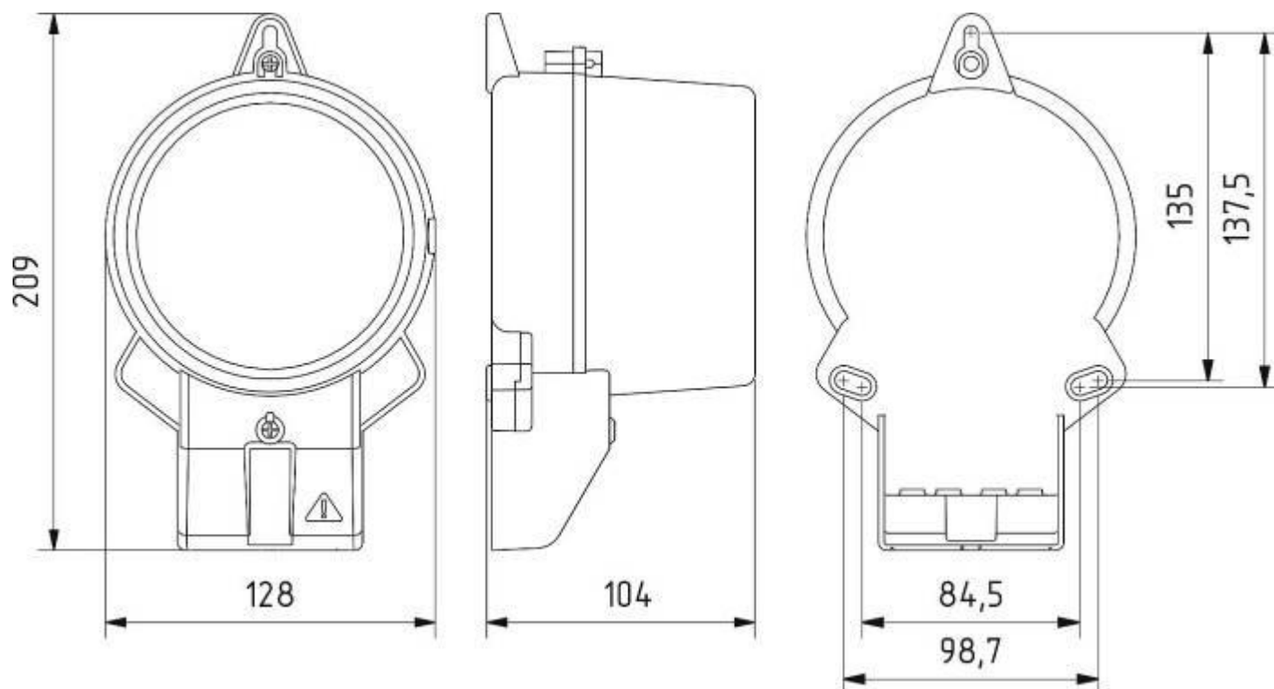
Рисунок В.4 – Тип корпуса W6
