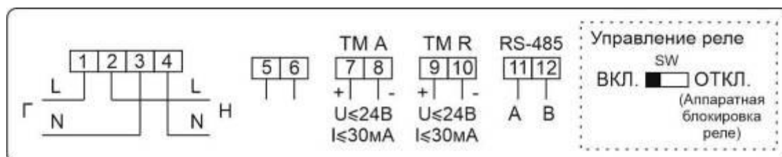
Рисунок Б.26 – Схема включения счетчиков в корпусах W3 с интерфейсом RS-485, с двумя (независимыми) дискретными выходами, настроенными как телеметрический выход активной энергии (ТМ А) и реактивной энергии (ТМ R) и аппаратной блокировкой встроенного реле управления нагрузкой (с помощью микропереключателя)
