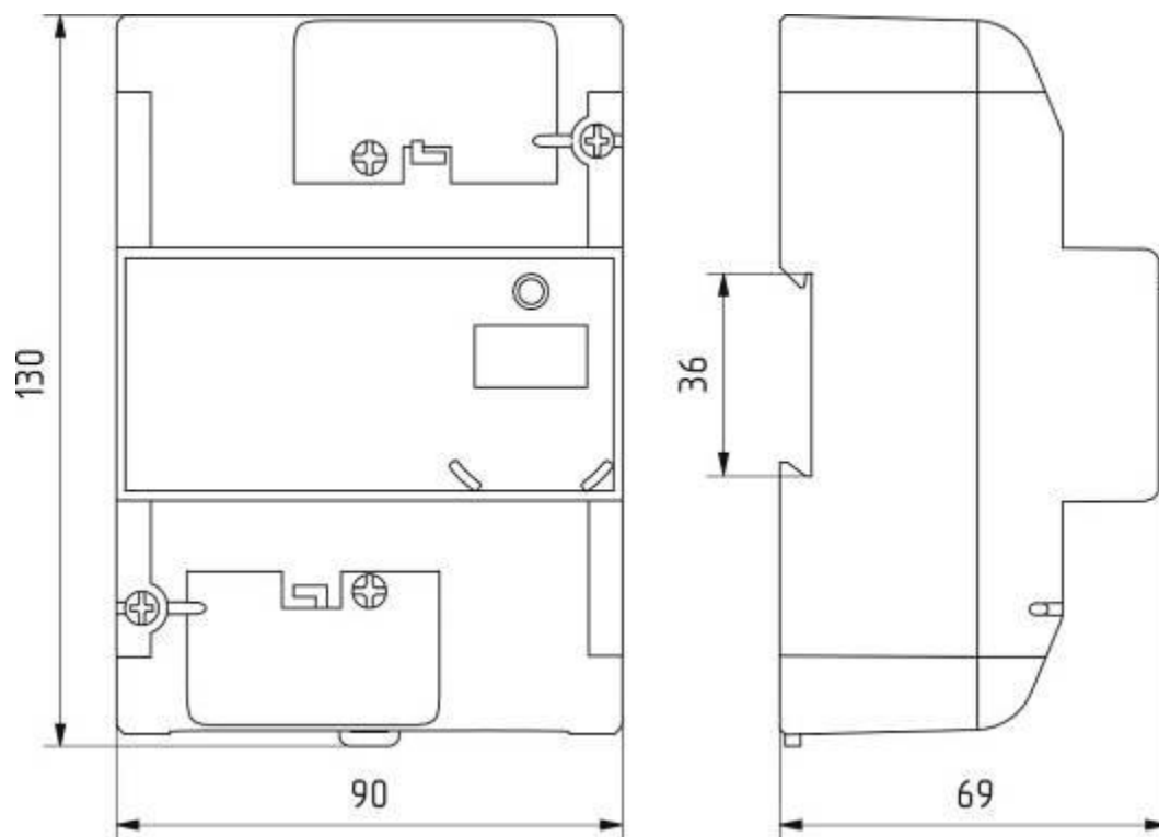
Рисунок В.7 – Тип корпуса D1
