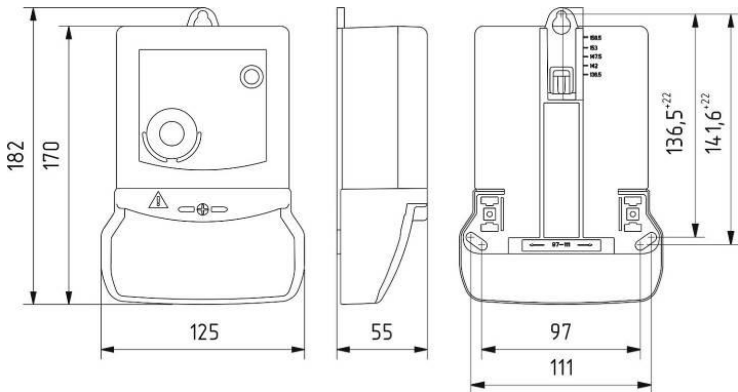
Рисунок В.2 – Тип корпуса W2
