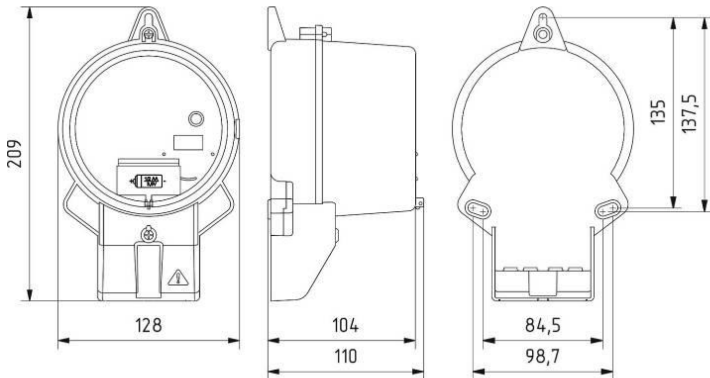
Рисунок В.5 – Тип корпуса W6b
