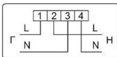
Рисунок Б.7 – Схема включения счетчиков в корпусах D5
