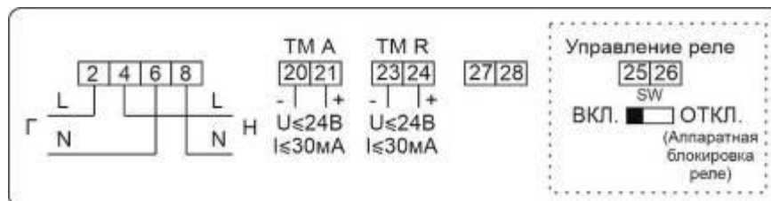
Рисунок Б.5 – Схема включения счетчиков в корпусах D1, D4 с двумя (независимыми) дискретными выходами, настроенными как телеметрический выход активной энергии (TM A) и реактивной энергии (TM R) и аппаратной блокировкой встроенного реле управления нагрузкой (с помощью микропереключателя)
