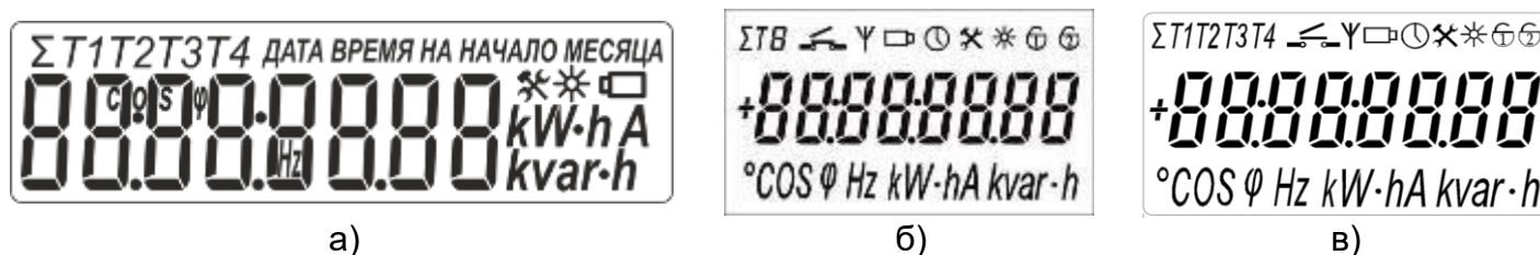
Рисунок 3.1 – Режим теста ЖКИ счетчика
