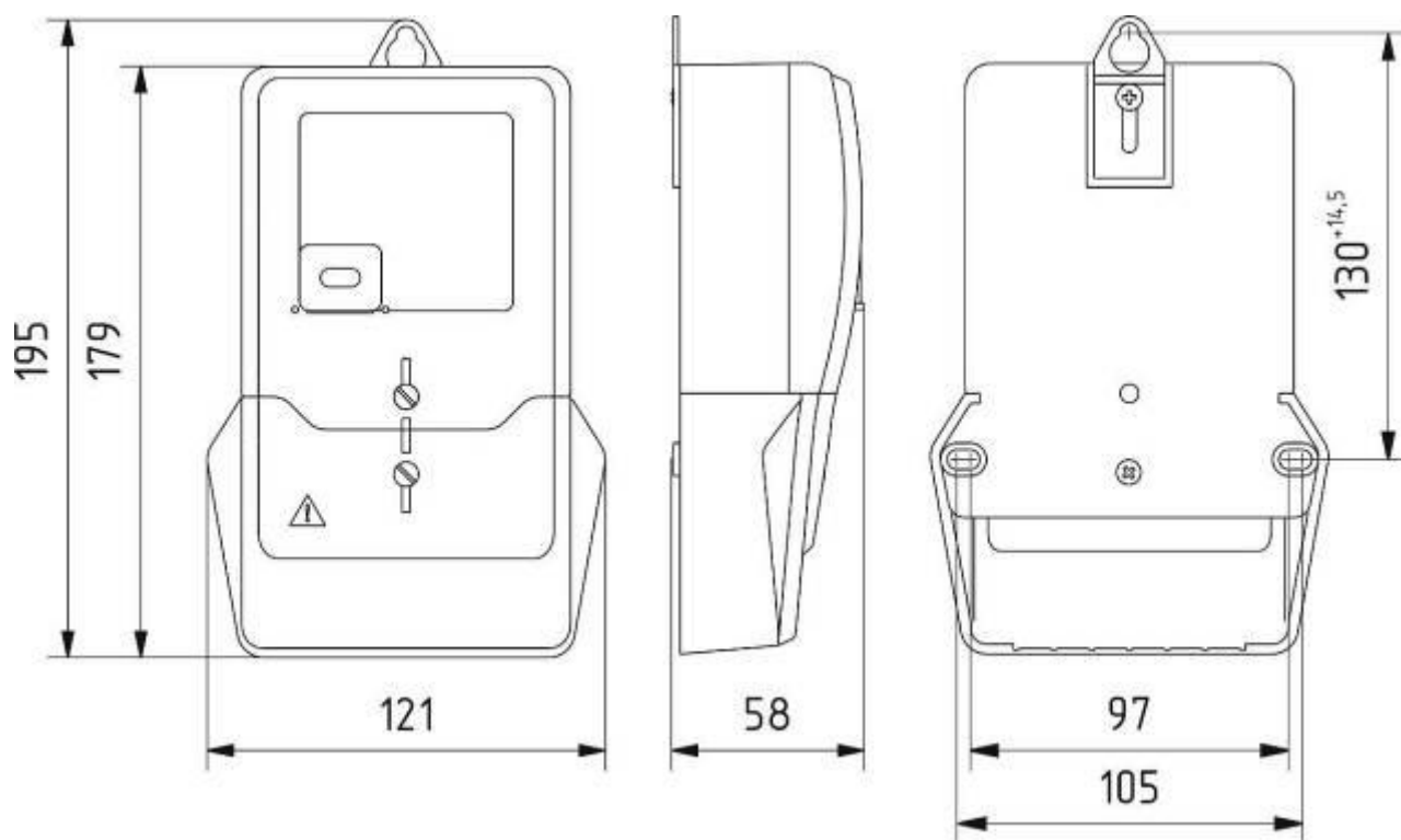
Рисунок В.1 – Тип корпуса W1
