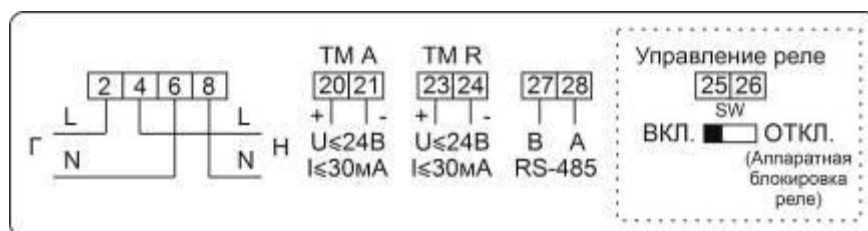
Рисунок Б.6 – Схема включения счетчиков в корпусах D1, D4 с двумя (независимыми) дискретными выходами, настроенными как телеметрический выход активной энергии (ТМ А) и реактивной энергии (ТМ R) и интерфейсом RS-485 и аппаратной блокировкой встроенного реле управления нагрузкой (с помощью микропереключателя)
