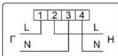
Рисунок Б.16 – Схема включения счетчиков в корпусах W2
