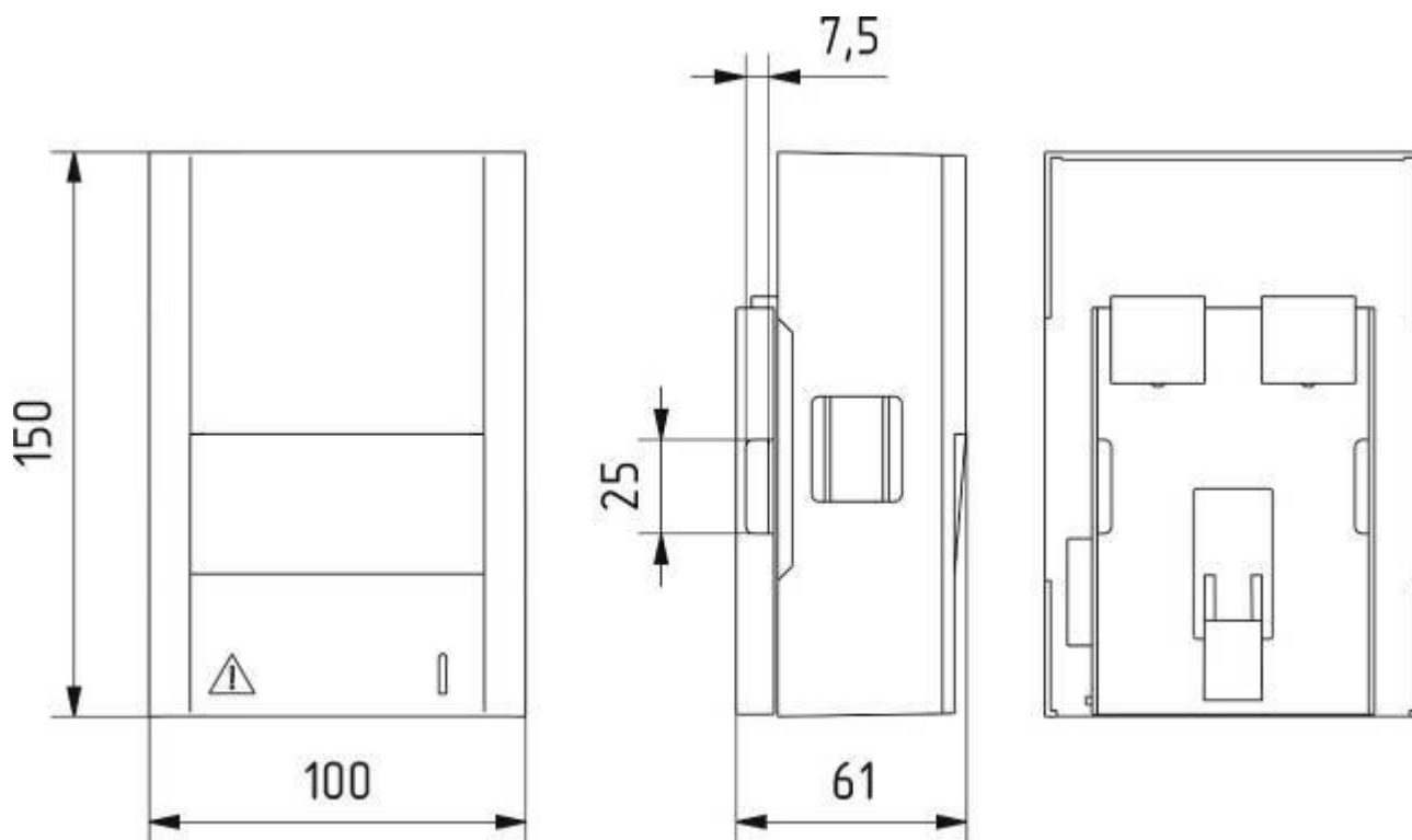
Рисунок В.15 – Тип корпуса SP2 с переходной пластиной, позволяющей осуществлять монтаж на опору ВЛ-0,4 кВ
