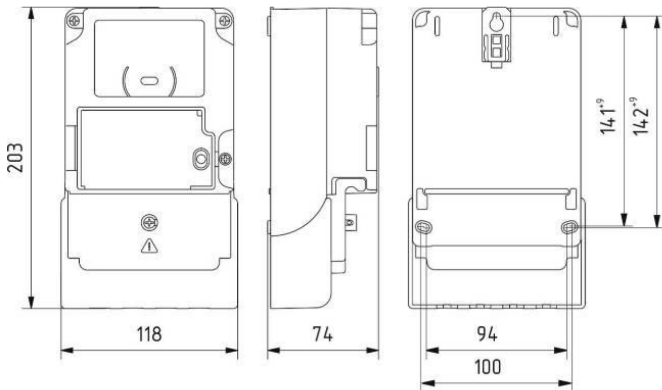
Рисунок В.3 – Тип корпуса W3
