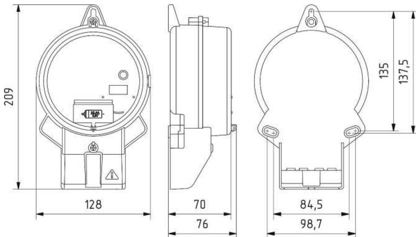
Рисунок В.6 – Тип корпуса W9
