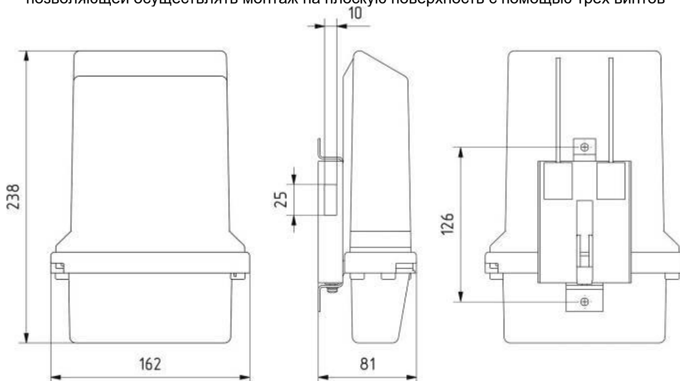
Рисунок В.14 – Тип корпуса SP1 с переходной пластиной, позволяющей осуществлять монтаж на опору ВЛ-0,4 кВ
