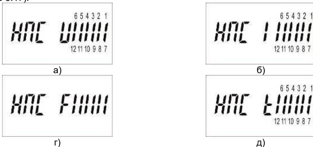
Рисунок 3.17 – Режимы индикации параметров качества сети
