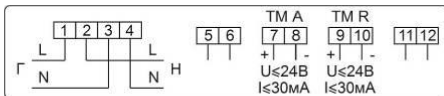
Рисунок Б.21 – Схема включения счетчиков в корпусах W3 с двумя (независимыми) дискретными выходами, настроенными как телеметрический выход активной энергии (TM A) и реактивной энергии (TM R)
