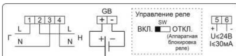
Рисунок Б.40 – Схема включения счетчиков в корпусе SP3 с одним дискретным выходом, настроенным как телеметрический выход (ТМ), разъёмом для подключения дополнительной сменной батарейки (GB1) и аппаратной блокировкой встроенного реле управления нагрузкой (с помощью микропереключателя)
