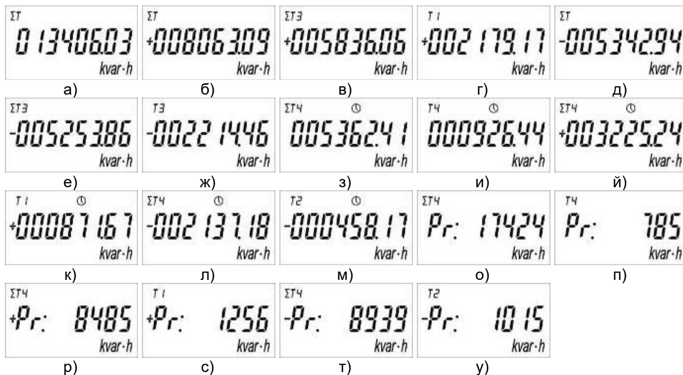
Рисунок 3.12 – Программируемые режимы индикации счетчика
