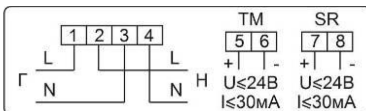
Рисунок Б.30 – Схема включения счетчиков в корпусах W6, W6b, W9 с двумя (независимыми) дискретными выходами, один из которых настроен как телеметрический выход (TM), а второй как реле сигнализации (SR)
