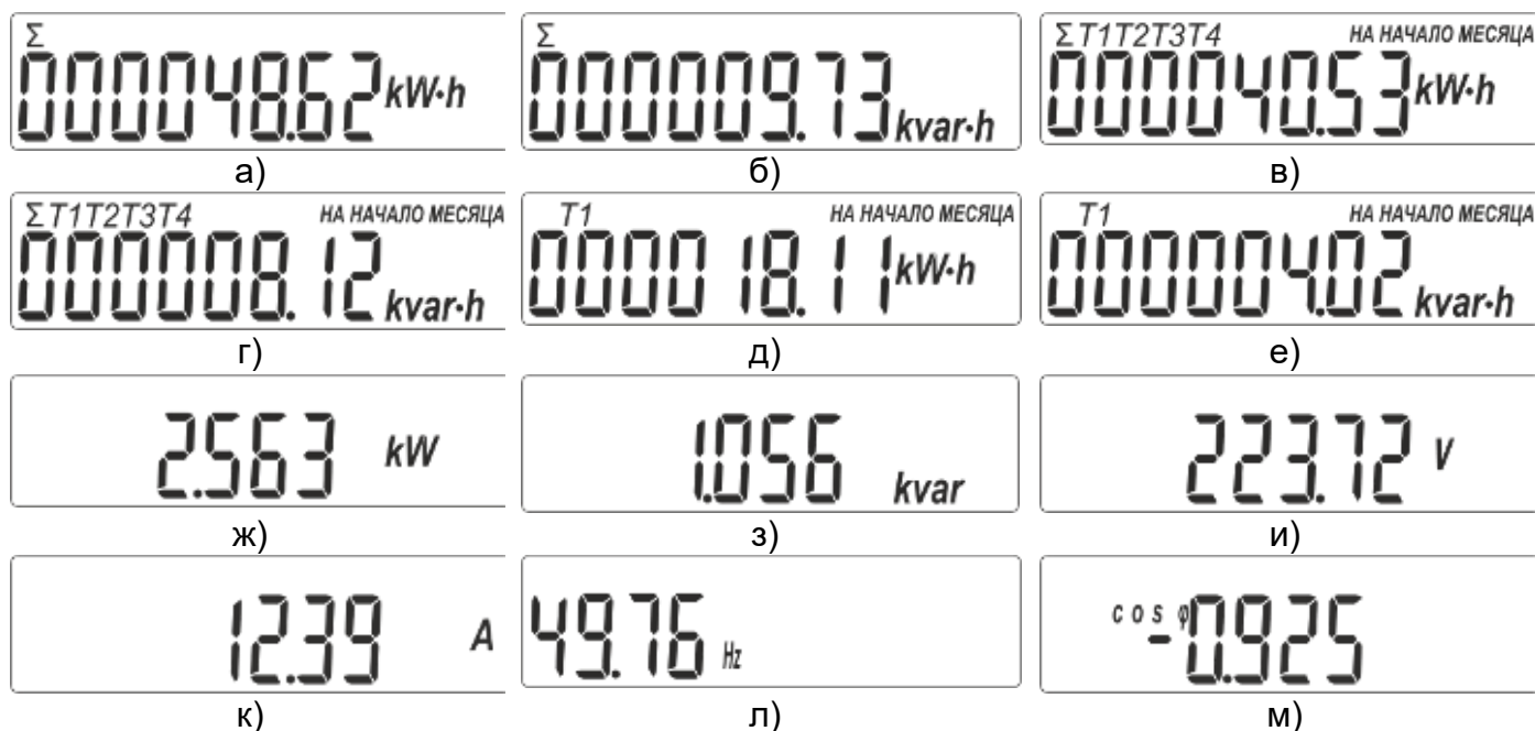
Рисунок 3.9 – Программируемые режимы индикации счетчика
