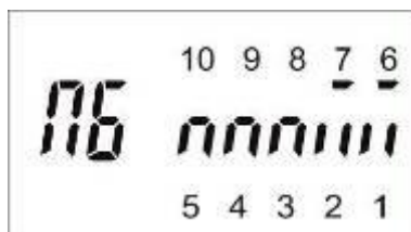
Рисунок 3.15 – Режимы индикации состояния электронных пломб счетчика
