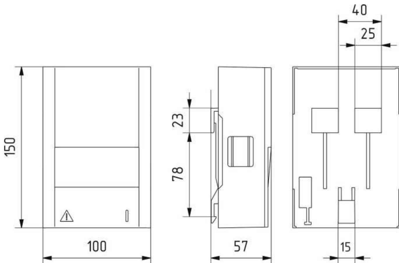
Рисунок В.11 – Тип корпуса SP2
