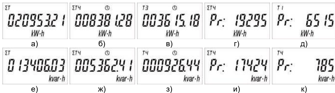
Рисунок Ж.4 – Программируемые режимы индикации счетчика
