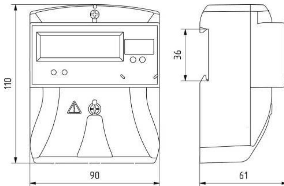
Рисунок В.9 – Тип корпуса D5
