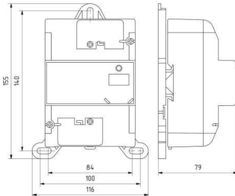
Рисунок В.13 – Тип корпуса D1 с переходной пластиной, позволяющей осуществлять монтаж на плоскую поверхность с помощью трех винтов
