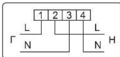
Рисунок Б.41 – Схема включения счетчиков в корпусах SP2
