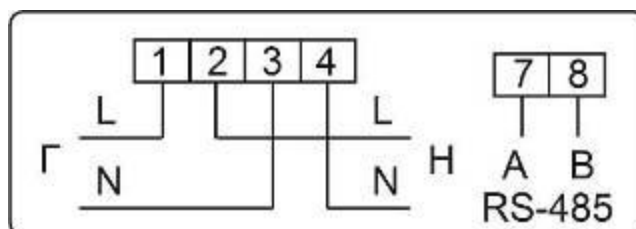
Рисунок Б.31 – Схема включения счетчиков в корпусах W6, W6b, W9 с интерфейсом RS-485
