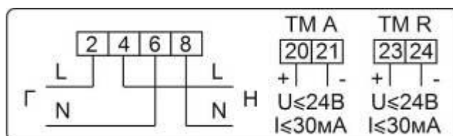
Рисунок Б.2 – Схема включения счетчиков в корпусах D1, D4 с двумя (независимыми) дискретными выходами, настроенными как телеметрический выход активной энергии (TM A) и реактивной энергии (TM R)
