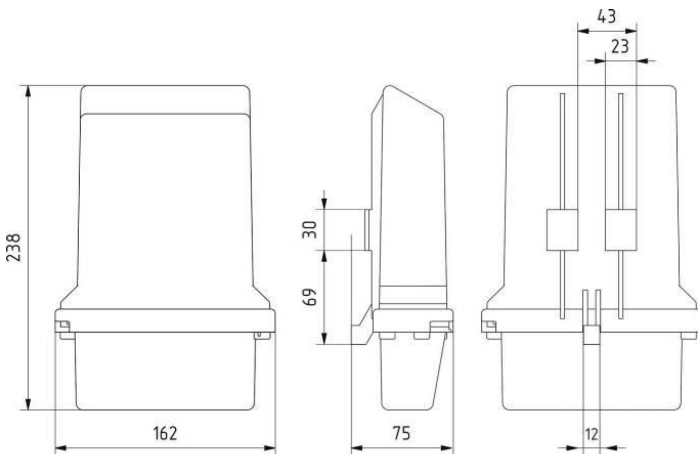
Рисунок В.10 – Тип корпуса SP1
