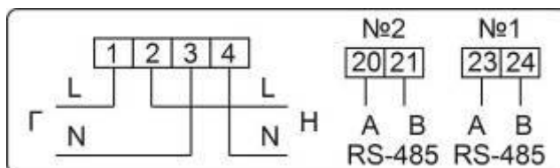
Рисунок Б.20 – Схема включения счетчиков в корпусах W2 с двумя (независимыми) интерфейсами RS-485
