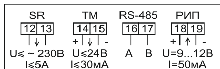
Рисунок Б.20 – Схема включения сигнальных цепей счетчиков в корпусе W31 с интерфейсом RS-485, с двумя (независимыми) дискретными выходами, один из которых настроен как телеметрический выход (TM), а второй как реле сигнализации (SR) с нагрузочной способностью 5А переменного тока и коммутируемым напряжением не более 230 В переменного напряжения и входом для подключения резервного источника питания
