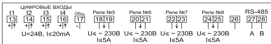
Рисунок Б.41 – Схема включения сигнальных цепей счетчиков в корпусе W32 с интерфейсом RS-485, с четырьмя (независимыми) дискретными выходами и с четырьмя дискретными входами (с одним общим проводом)
