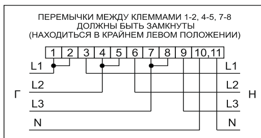
Рисунок Б.7 – Схема включения счетчиков в корпусе W31 непосредственного включения на измерительных элементах трансформаторах тока
