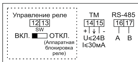
Рисунок Б.23 – Схема включения сигнальных цепей счетчиков в корпусе W31 непосредственного включения с интерфейсом RS-485, с одним дискретным выходом, настроенным как телеметрический выход (TM) и аппаратной блокировкой встроенного реле управления нагрузкой (с помощью микропереключателя)
