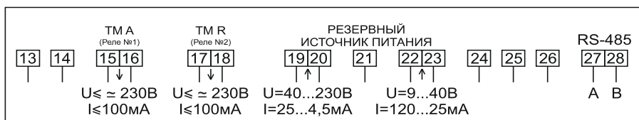
Рисунок Б.38 – Схема включения сигнальных цепей счетчиков в корпусе W32 с интерфейсом RS-485, с двумя (независимыми) дискретными выходами, с двумя входами для подключения резервного источника питания в диапазоне от 9 до 40 В и от 40 до 230 В (вариант 2)
