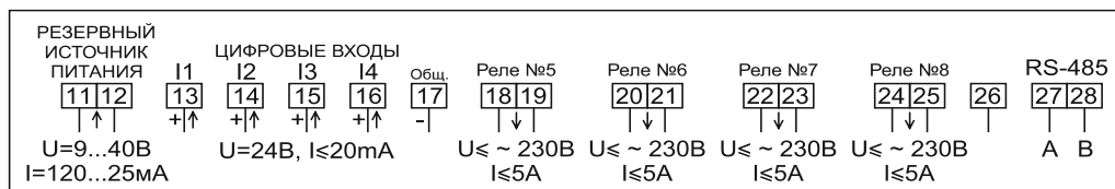
Рисунок Б.42 – Схема включения сигнальных цепей счетчиков в корпусе W32 трансформаторного включения, с интерфейсом RS-485, с четырьмя (независимыми) дискретными выходами и с четырьмя дискретными входами (с одним общим проводом), с одним входом для подключения резервного источника питания в диапазоне от 9 до 40 В
