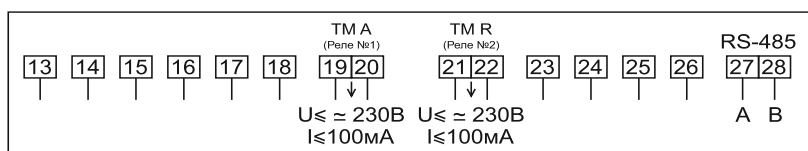
Рисунок Б.32 – Схема включения сигнальных цепей счетчиков в корпусе W32 с интерфейсом RS-485, с двумя (независимыми) дискретными выходами (вариант 1)
