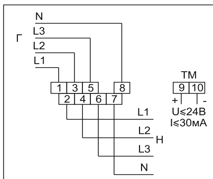
Рисунок Б.58 – Схема включения счетчиков в корпусах SP31 с одним дискретным выходом, настроенным как телеметрический выход (ТМ)
