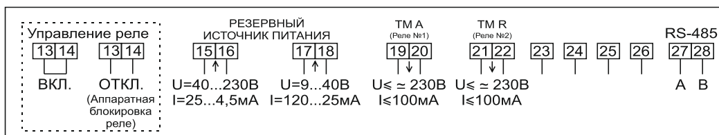
Рисунок Б.48 – Схема включения сигнальных цепей счетчиков в корпусе W32 непосредственного включения с интерфейсом RS-485, с двумя (независимыми) дискретными выходами, с двумя входами для подключения резервного источника питания в диапазоне от 9 до 40 В и от 40 до 230 В, аппаратной блокировкой встроенного реле управления нагрузкой (с помощью клеммника)
