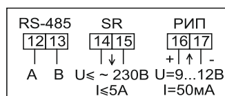
Рисунок Б.19 – Схема включения сигнальных цепей счетчиков в корпусе W31 с интерфейсом RS-485, с одним дискретным выходом, настроенным как реле сигнализации (SR) с нагрузочной способностью 5А переменного тока и коммутируемым напряжением не более 230 В переменного напряжения, и входом для подключения резервного источника питания
