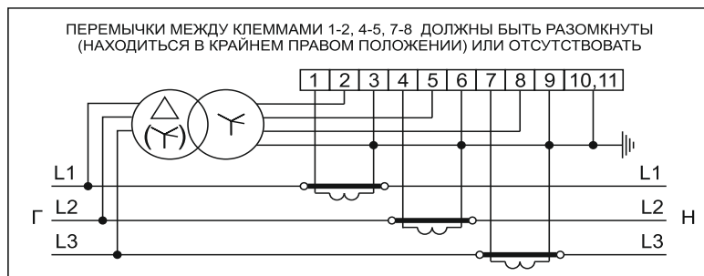
Рисунок Б.3 – Схема включения счетчиков в корпусах D33 трансформаторного включения через три трансформатора напряжения и три трансформатора тока
