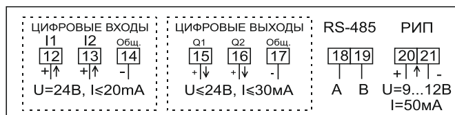
Рисунок Б.21 – Схема включения сигнальных цепей счетчиков в корпусе W31 с интерфейсом RS-485, с двумя дискретными входами (с одним общим проводом) и с двумя дискретными выходами (с одним общим проводом) и входом для подключения резервного источника питания
