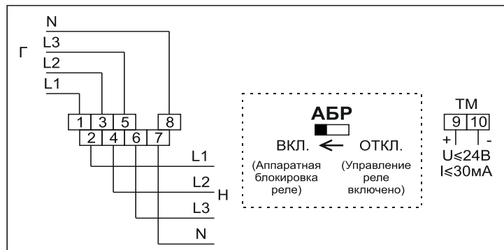
Рисунок Б.60 – Схема включения счетчиков в корпусах SP31 с одним дискретным выходом, настроенным как телеметрический выход (ТМ), и аппаратной блокировкой встроенного реле управления нагрузкой (с помощью микропереключателя)
