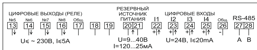
Рисунок Б.44 – Схема включения сигнальных цепей счетчиков в корпусе W32 с интерфейсом RS-485, с четырьмя дискретными выходами (с одним общим проводом) и с четырьмя дискретными входами (с одним общим проводом), с одним входом для подключения резервного источника питания в диапазоне от 9 до 40 В
