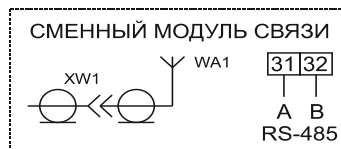
Рисунок Б.63 – Схема включения сигнальных цепей сменного модуля связи счетчиков в корпусах W32 с GSM/GPRS-модулем с дополнительным интерфейсом RS485 для подключения дополнительных устройств
