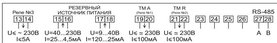
Рисунок Б.39 – Схема включения сигнальных цепей счетчиков в корпусе W32 с интерфейсом RS-485, с тремя (независимыми) дискретными выходами с двумя входами для подключения резервного источника питания в диапазоне от 9 до 40 В и от 40 до 230 В (вариант 1)
