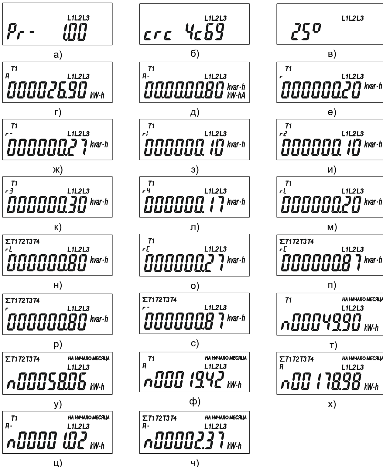
Рисунок 3.11 – Программируемые режимы индикации счетчика
