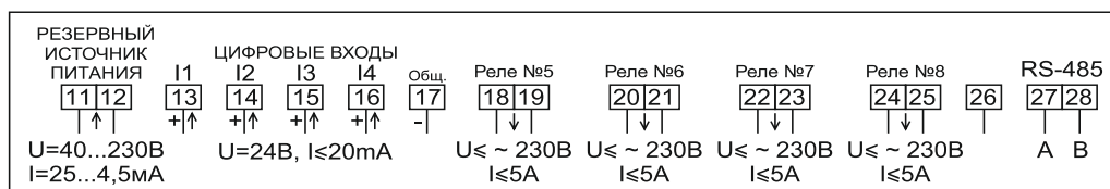
Рисунок Б.43 – Схема включения сигнальных цепей счетчиков в корпусе W32 трансформаторного включения, с интерфейсом RS-485, с четырьмя (независимыми) дискретными выходами и с четырьмя дискретными входами (с одним общим проводом), с одним входом для подключения резервного источника питания в диапазоне от 40 до 230 В
