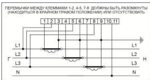
10-ти проводная схема
