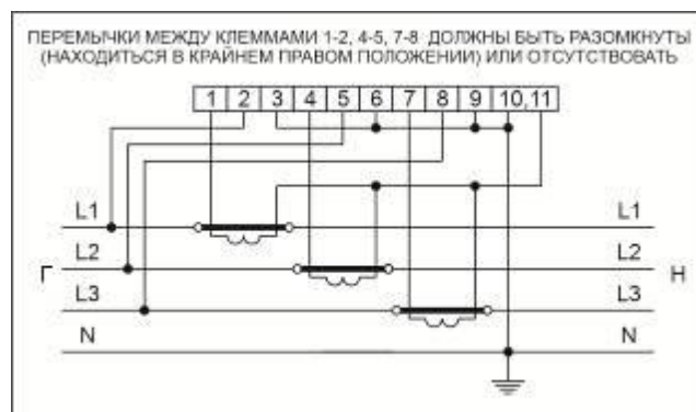
8-ми проводная схема
