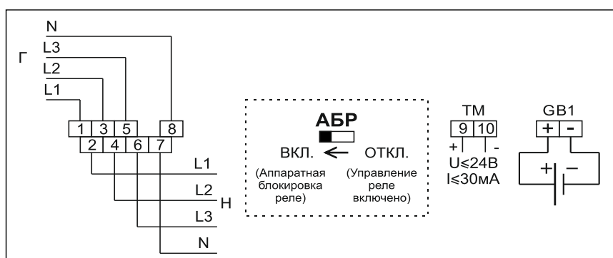
Рисунок Б.61 – Схема включения счетчиков в корпусах SP31 с одним дискретным выходом, настроенным как телеметрический выход (ТМ), разъемом для подключения дополнительной сменной батарейки (GB1) и аппаратной блокировкой встроенного реле управления нагрузкой (с помощью микропереключателя)
