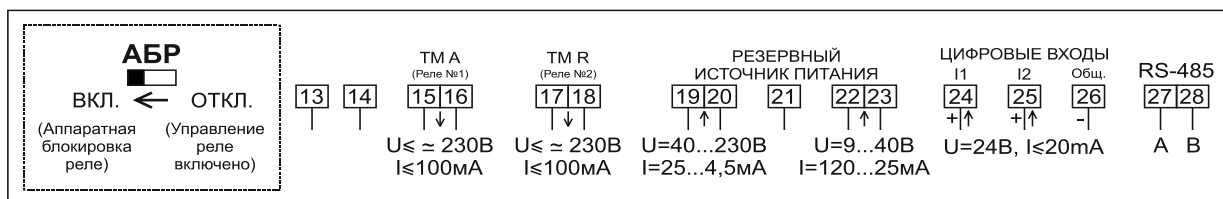
Рисунок Б.53 – Схема включения сигнальных цепей счетчиков в корпусе W32 непосредственного включения с интерфейсом RS-485, с двумя (независимыми) дискретными выходами, с двумя дискретными входами (с одним общим проводом), с двумя входами для подключения резервного источника питания в диапазоне от 9 до 40 В и от 40 до 230 В, аппаратной блокировкой встроенного реле управления нагрузкой (с помощью микропереключателя)
