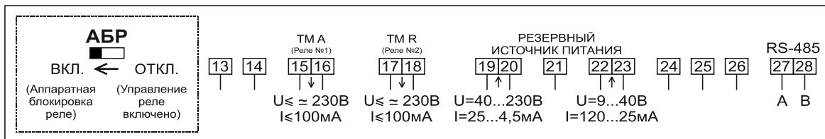
Рисунок Б.51 – Схема включения сигнальных цепей счетчиков в корпусе W32 непосредственного включения с интерфейсом RS-485, с двумя (независимыми) дискретными выходами, с двумя входами для подключения резервного источника питания в диапазоне от 9 до 40 В и от 40 до 230 В, аппаратной блокировкой встроенного реле управления нагрузкой (с помощью микропереключателя)
