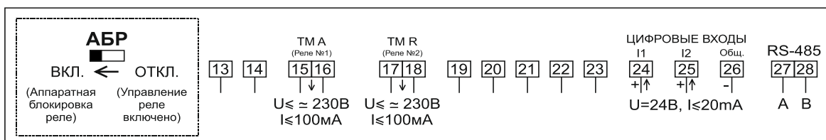
Рисунок Б.52 – Схема включения сигнальных цепей счетчиков в корпусе W32 непосредственного включения с интерфейсом RS-485, с двумя (независимыми) дискретными выходами и с двумя дискретными входами (с одним общим проводом), аппаратной блокировкой встроенного реле управления нагрузкой (с помощью микропереключателя)
