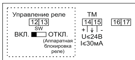
Рисунок Б.22 – Схема включения сигнальных цепей счетчиков в корпусе W31 непосредственного включения с одним дискретным выходом, настроенным как телеметрический выход (TM) и аппаратной блокировкой встроенного реле управления нагрузкой (с помощью микропереключателя)
