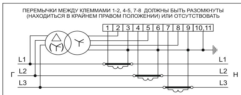
Рисунок Б.9 – Схема включения счетчиков в корпусах W31 трансформаторного включения через три трансформатора напряжения и три трансформатора тока
