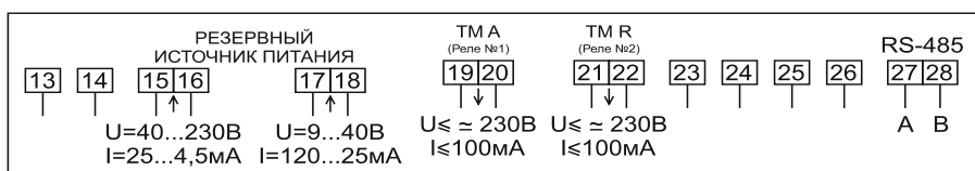
Рисунок Б.37 – Схема включения сигнальных цепей счетчиков в корпусе W32 с интерфейсом RS-485, с двумя (независимыми) дискретными выходами, с двумя входами для подключения резервного источника питания в диапазоне от 9 до 40 В и от 40 до 230 В (вариант 1)
