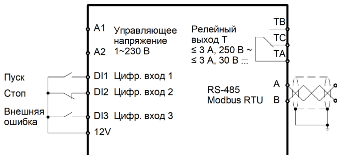
Рис.5а. Подключение клемм управления серии SBIM мощностью до 15 кВт
