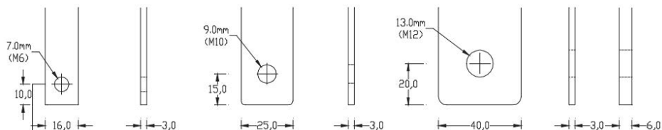
2T1, 4T2, 6T3 Типоразмер 3
