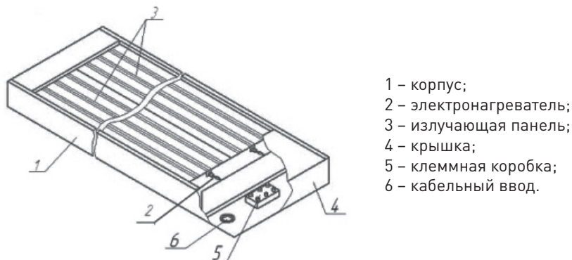
Рис.1. Обогреватель инфракрасный.
