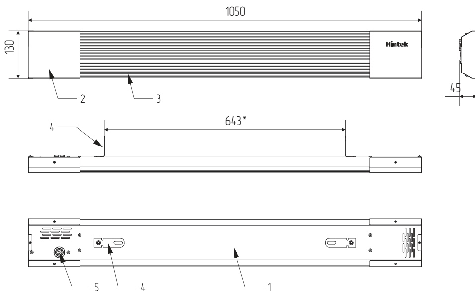
Рисунок 2. Габаритный чертёж и элементы конструкции инфракрасного обогревателя IC 08 IP54.
