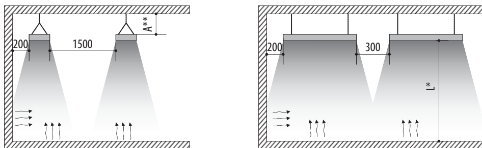
Рисунок 5. Минимальные расстояния от обогревателя до других поверхностей (мм).
