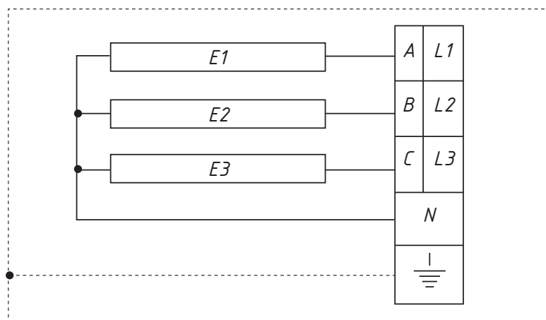
Рис. 5. Схема подключения обогревателей IO-05, IO-10, IO-15, IO-20, IO-30
