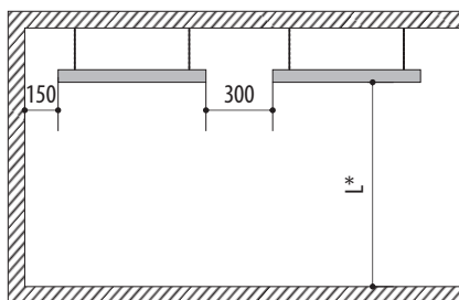
Рисунок 3. Минимальные расстояния от обогревателя до других поверхностей (мм).
