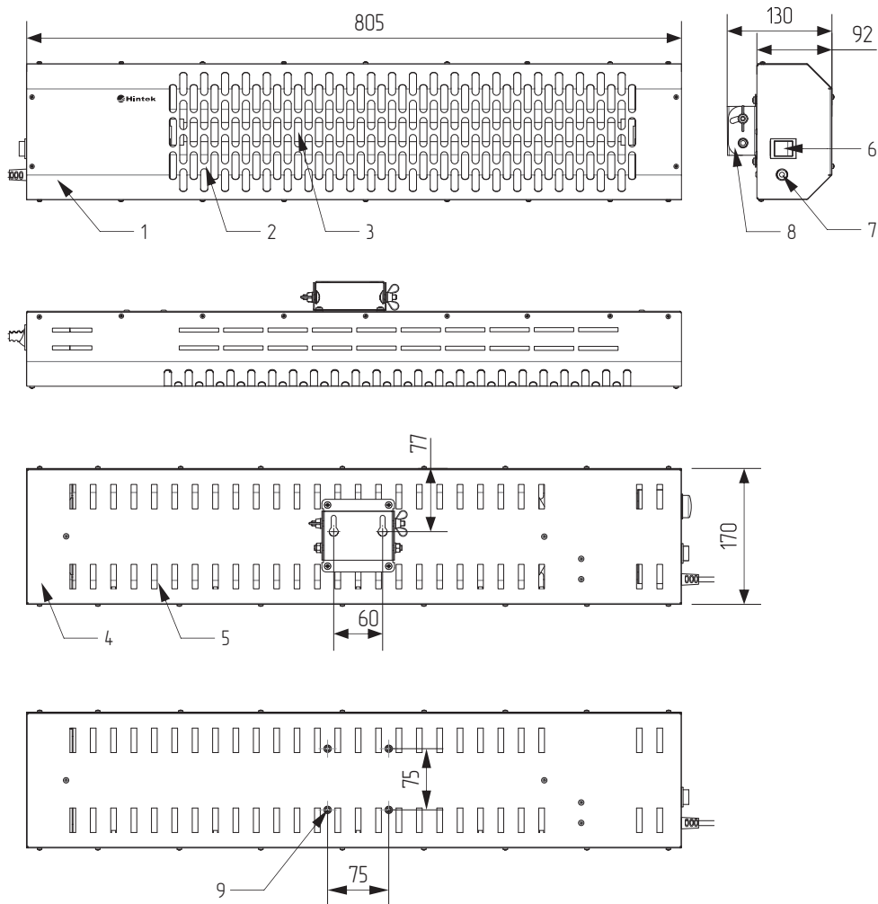
Рисунок 2. Габаритный чертёж и элементы конструкции электрического обогревателя Unicum-1500, Unicum-2000.
