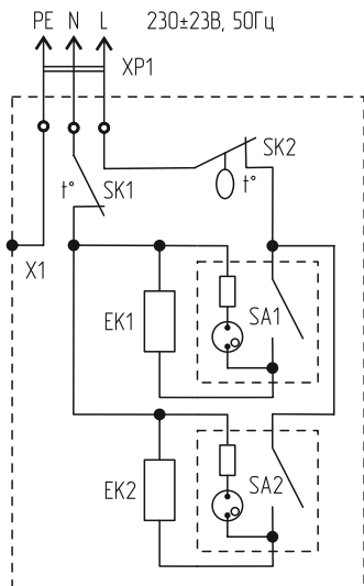
Рисунок 5. Электрическая схема конвектора (А – Standart 500M, Standart 1000M, Б – Standart 1500M, Standart 2000M, Standart 2500M)
