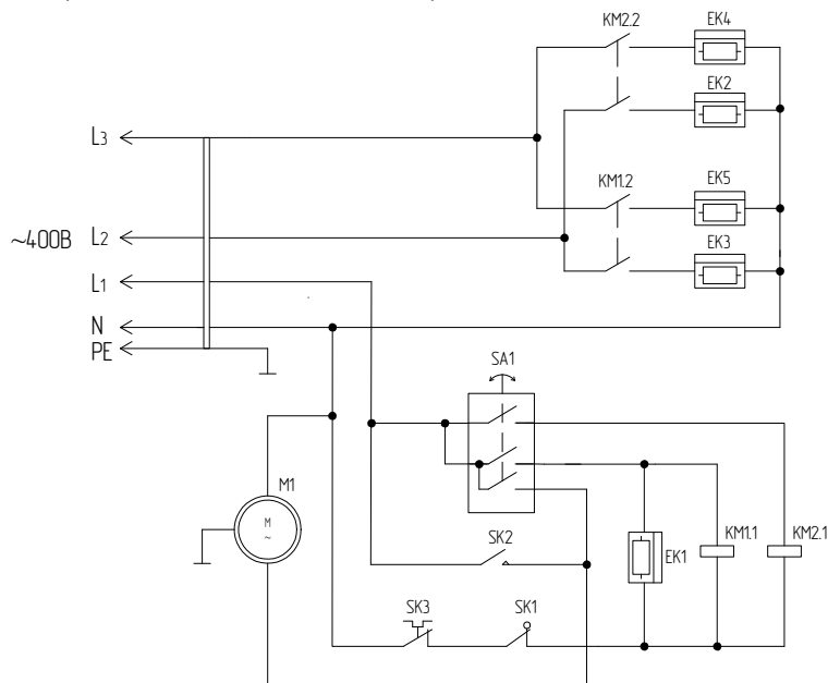
Электрическая схема тепловентилятора TP-153805
