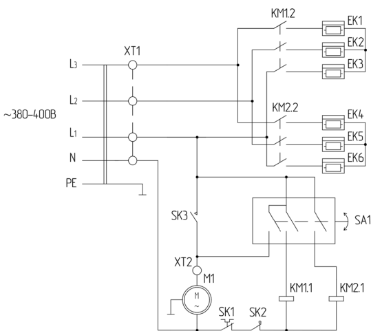
Рис. 2 Схема электрическая тепловентилятора T-24380S
