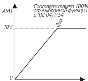
Рисунок 5.3.11.1 АМ1-5, сигнал выход 0 ~ 10 В
