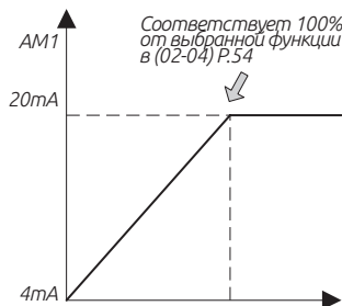
5.3.11.3. Выход АМ1-5, сигнал 4 ~ 20 мА
