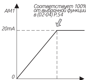
Рисунок 5.3.11.2. АМ1-5, сигнал 0 ~ 20 мА
