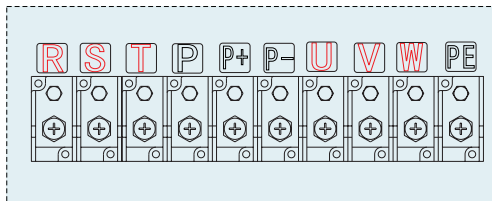
Рисунок 3-16. Схема силовых клемм ПТ мощностью 400-500 кВт
