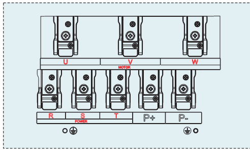
Рисунок 3-14. Схема силовых клемм ПТ мощностью 132-250 кВт
