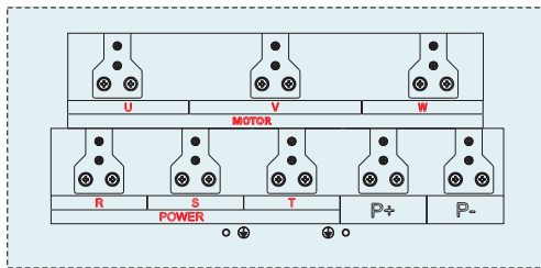
Рисунок 3-15. Схема силовых клемм ПТ мощностью 280-355 кВт
