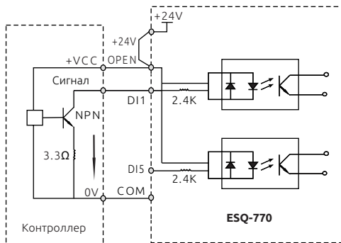
Рисунок 3-19. Подключение внешнего контроллера в режиме «Sink».
