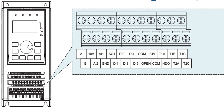
Рисунок 3.17.1 Клеммы управления 0.75-4 кВт
