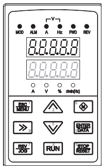
Рис. а отображение при подаче питания
