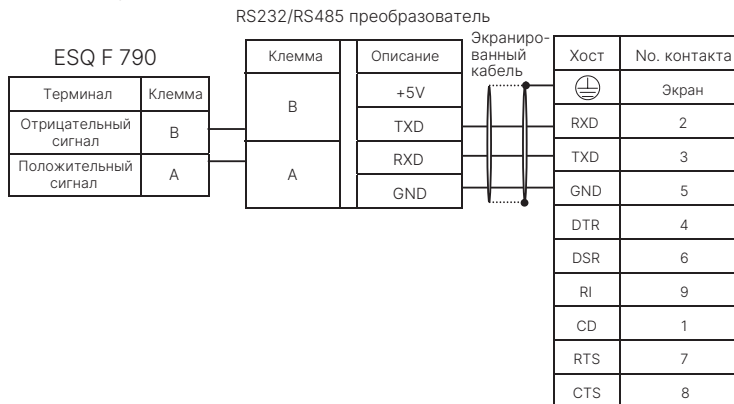
Рис. 3-18 Схема подключения через интерфейс RC485
