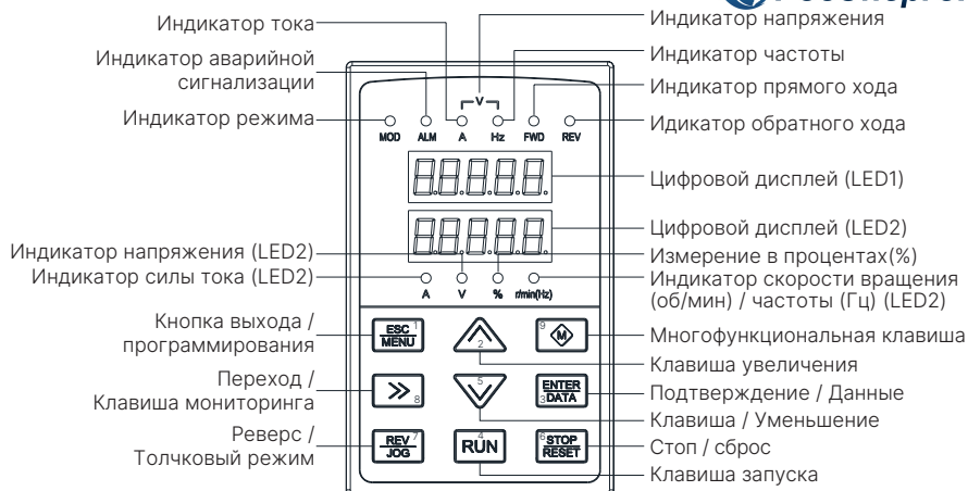
EN-LED16 Схема расположения клавиш Рис. 5-2 Устройство панели управления
