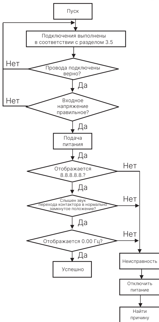
Рис. 5-12 Порядок действий при включении питания
