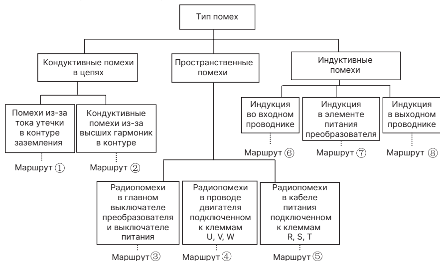
Рис.4-1 Типы помех
