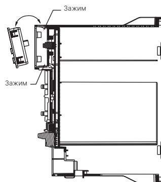
Fig. 3-3 Установка клавиатуры
