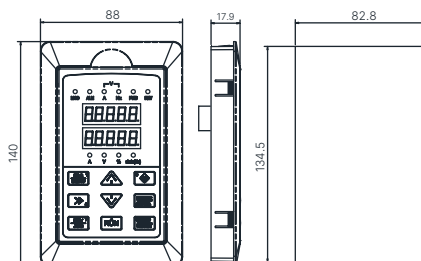
Рис. 2-5 EN-LED15 внешний вид и размеры отверстия клавиатуры
