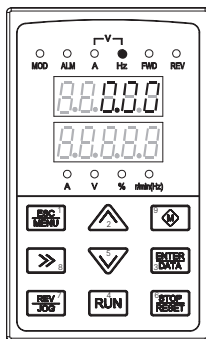
Рис. б Режим ожидания, отображение параметров режима ожидания
