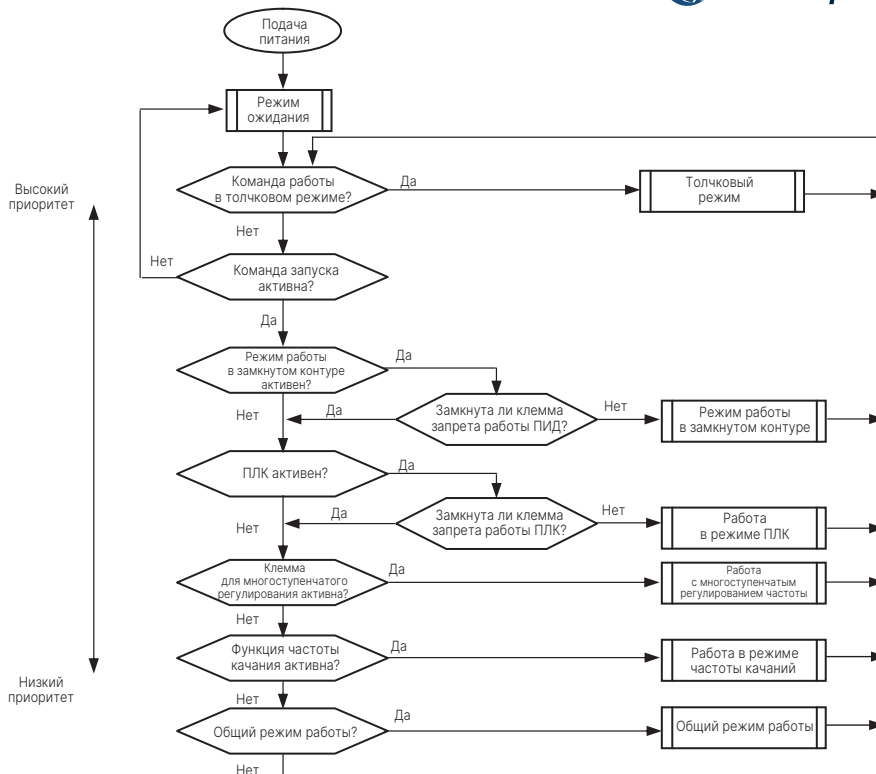
Рис. 5-1 Режимы работы
