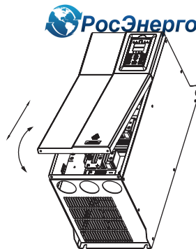
Рис. 3-5 Снятие и установка крышки
