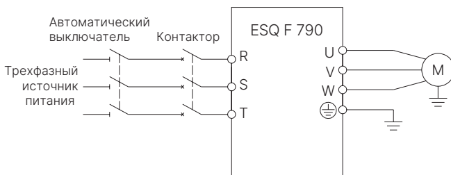
Рис. 3-7 Схема подключения силовой цепи
