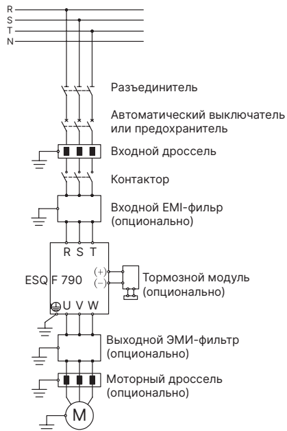
Fig. 3-8 Подключение преобразователя и дополнительных компонентов
