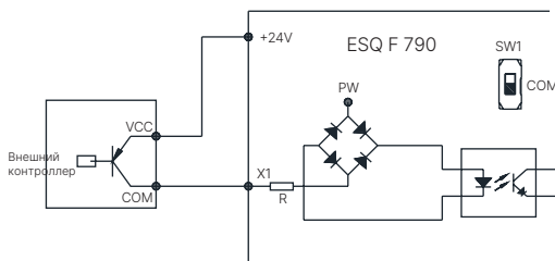
Рис. 3-15 Подключение встроенного источника питания 24 В в режиме «Приемник»
