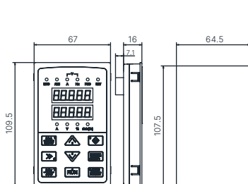
Рис. 2-5 EN-LED15 внешний вид и размеры отверстия клавиатуры
