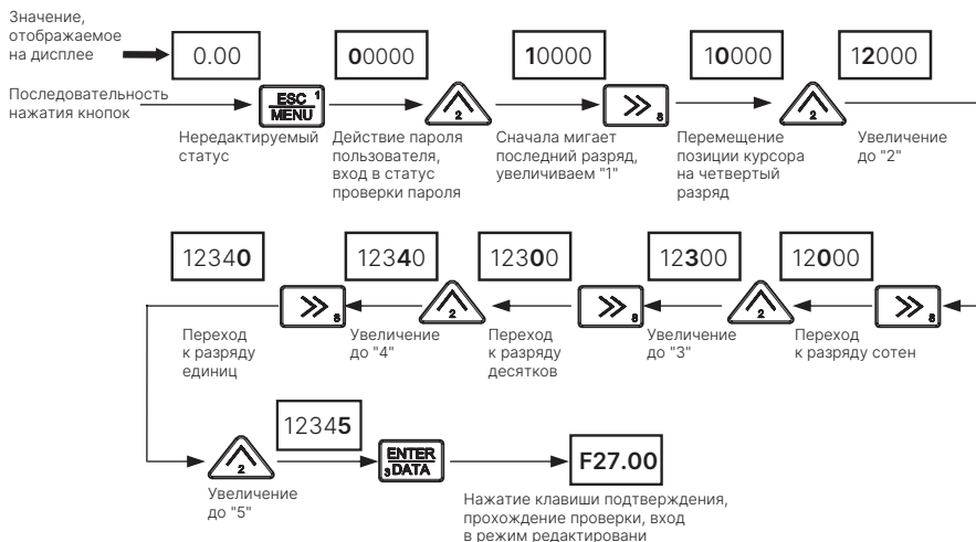
Рис. 5-11 Ввод пароля для перехода к операции с функциональным кодом
