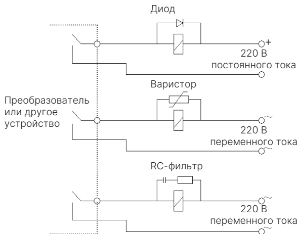
Рис. 4-3 Требования к установке электронных устройств с электромагнитным переключателем
