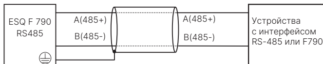
Рис. 3-17 Схема подключения терминала связи
