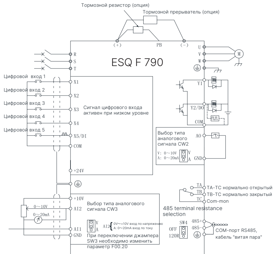
Рис. 3-9 Схема электрических подключений
