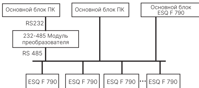
Рис. В-1 Схематическая диаграмма способа организации сети
