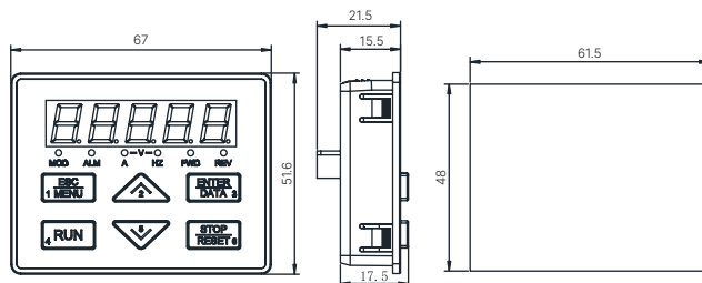
Рис. 2-5 EN-LED15 внешний вид и размеры отверстия клавиатуры
