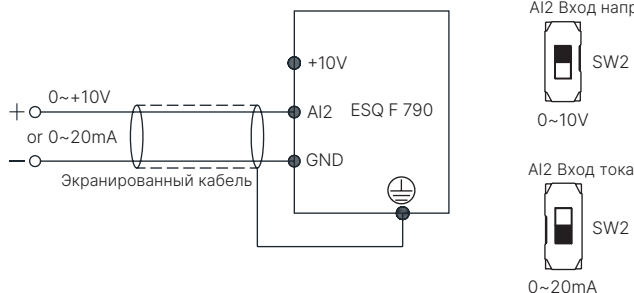
Рис. 3-12 Схема подключения клеммы AI2
