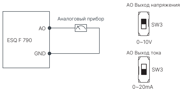
Рис. 3-13 Схема подключения клемм АО
