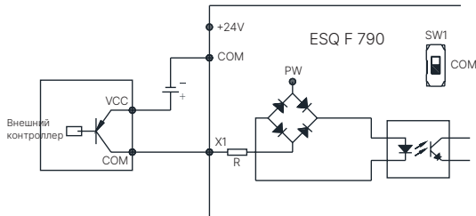
Рис. 3-16 Подключение к внешнему источнику питания в режиме «Источник»
