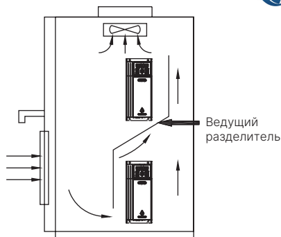
Рис. 3-2 Монтаж нескольких преобразователей
