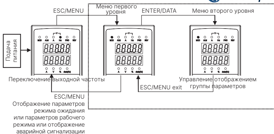
Рис. 5-5 Переключение статусов отображения на клавиатуре
