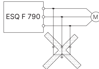
Рис. 1-2 Конденсатор на выходной стороне запрещен
