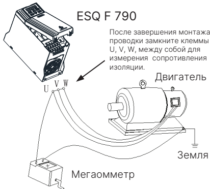
Рис. 1-1 Проверка изоляции мотора
