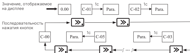
Рис. 5-7 Пример операции отображения параметров в режиме ожидания
