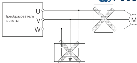
Рис. 3-6 Запрещено использовать контактор и фильтрующий конденсатор
