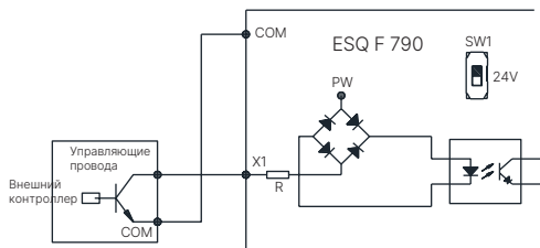
Рис. 3-14 Подключение встроенного источника питания 24 В в режиме «Источник»
