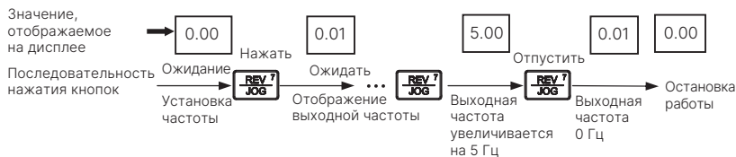
Рис. 5-10 Пример операции толчкового режима
