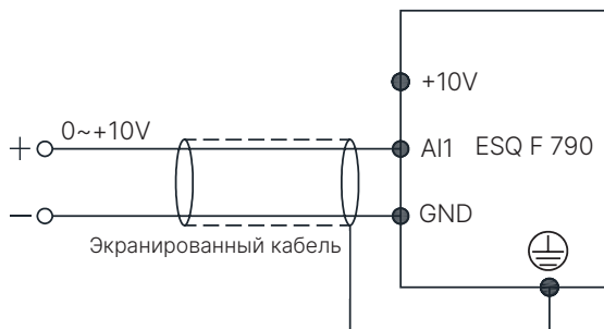
Рис. 3-11 Схема подключения клеммы AI1
