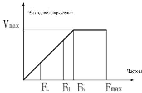
Рис. 7-1 Схема определения параметров частоты
