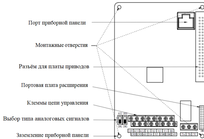
Рис. 3-16 Плата управления
