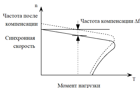
Рис. 6-11 Автоматическая компенсация скольжения
