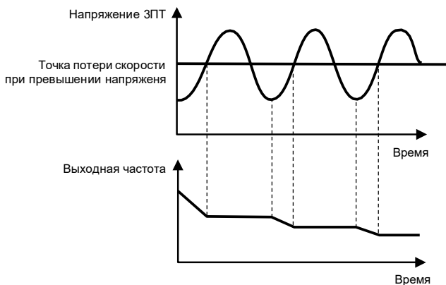
Рисунок 6.19 – Иллюстрация работы защиты от перенапряжения
