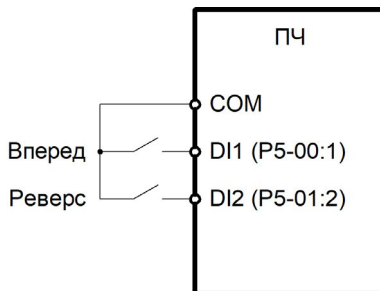
Рисунок 6.9 – Схема двухпроводного подключения 1
