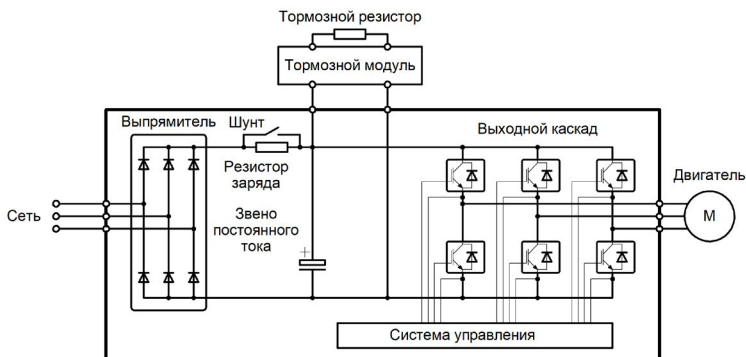
Рисунок 2.2 - Принципиальная электрическая схема для трехфазных моделей INPRIME MX с внешним тормозным модулем
