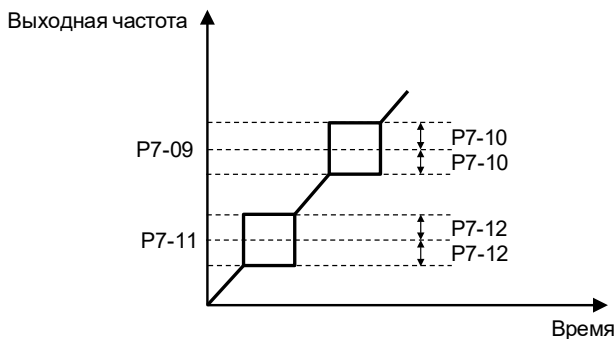
Рисунок 6.14 – Принцип работы функции скачкообразной перестройки
