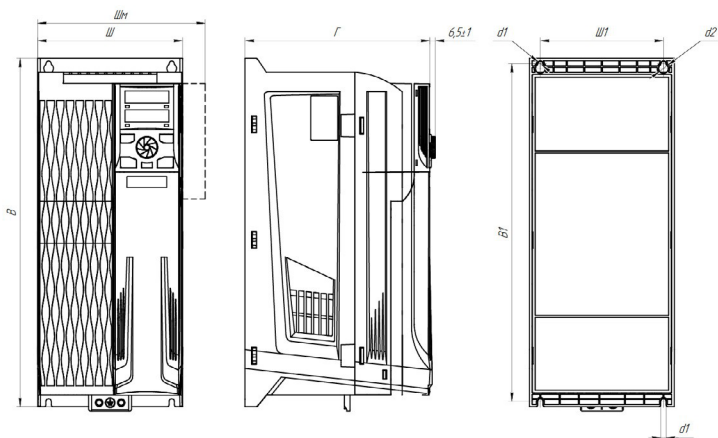
Рисунок 2.5 – Габаритные и установочные размеры устройств серии INPRIME MX в пластмассовом корпусе (настенное исполнение), типоразмеры 1-4
