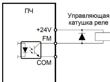
Рисунок 3.18 – Подключение к цифровому выходу с использованием внутреннего источника питания
