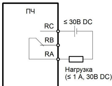
Рисунок 3.17 – Схема подключения нагрузки постоянного тока к релейному выходу
