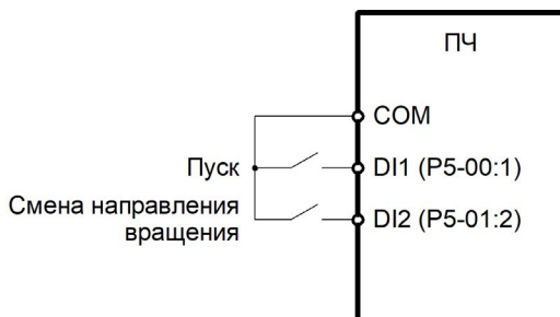
Рисунок 6.10 – Схема двухпроводного подключения 2
