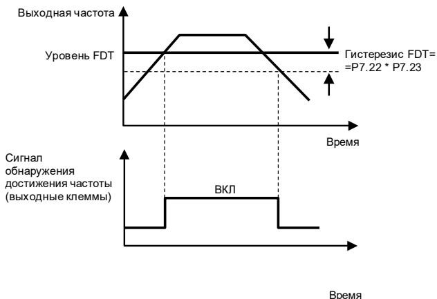
Рисунок 6.16 – Значение обнаружения выходной частоты
