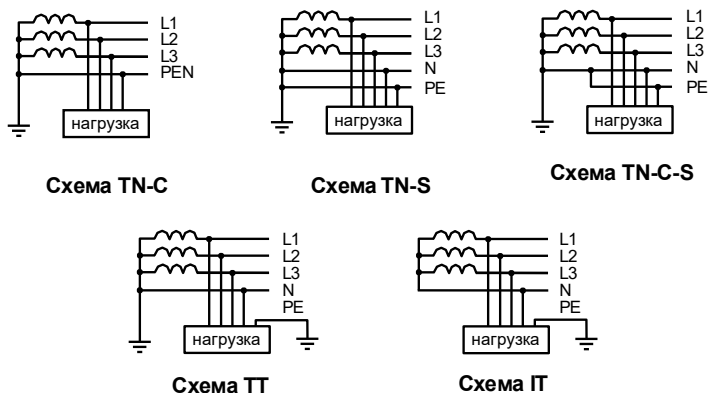
Рисунок 3.10 – Типы систем заземления
