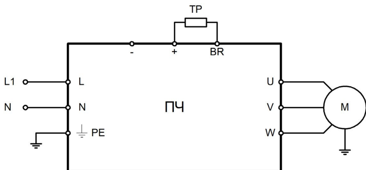
Рисунок 3.4 – Схема силовых подключений для моделей INPRIME MX-GY-3B
