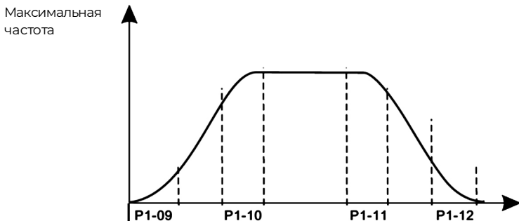
Рисунок 6.4 – S-образная кривая ускорения и замедления
