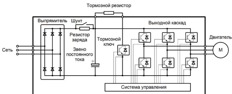
Рисунок 2.1 – Принципиальная электрическая схема для трехфазных моделей INPRIME MX со встроенным тормозным модулем
