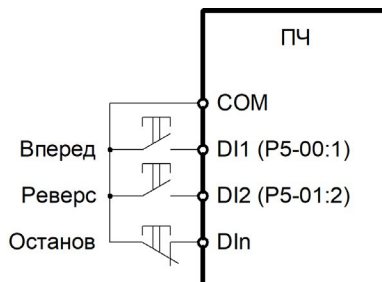
Рисунок 6.11 – Схема трехпроводного подключения 1
