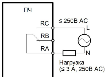
Рисунок 3.16 – Схема подключения нагрузки переменного тока к релейному выходу
