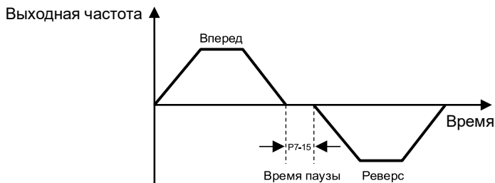
Рисунок 6.15 – Время паузы при смене направления вращения
