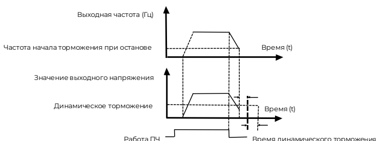
Рисунок 6.5 – Процесс торможения постоянным током
