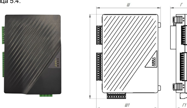
Рисунок 5.7 – Модуль INMX-Ecard
