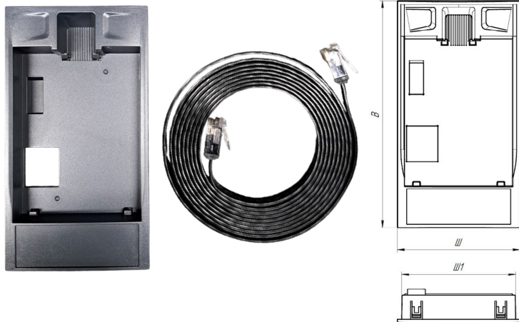
Рисунок 5.3 – Монтажный комплект INMX-MK и чертеж монтажной рамки INMX-MF
