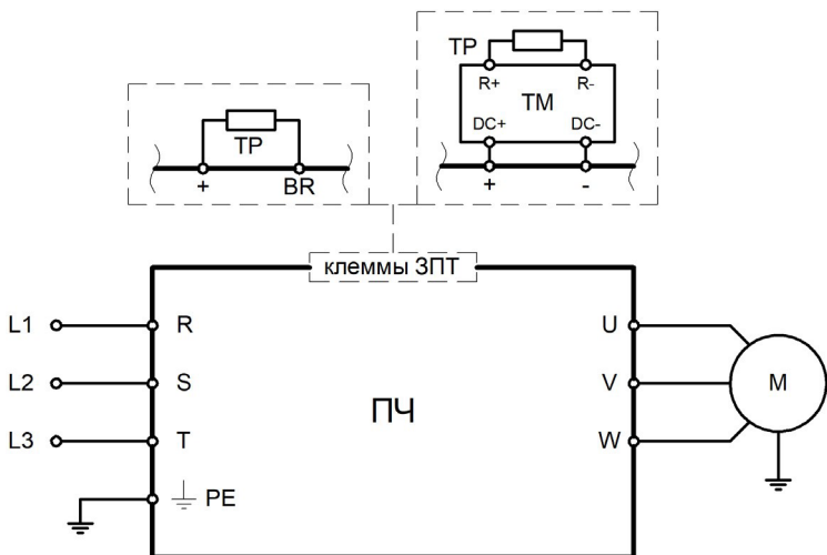
Рисунок 3.5 – Схема силовых подключений для моделей INPRIME MX-GY/PY-4B
