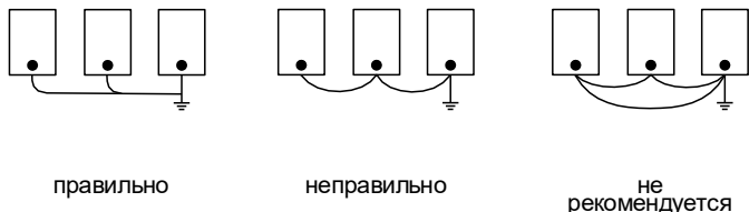
Рисунок 3.9 – Схематичное изображение образования петли с заземляющим проводом
