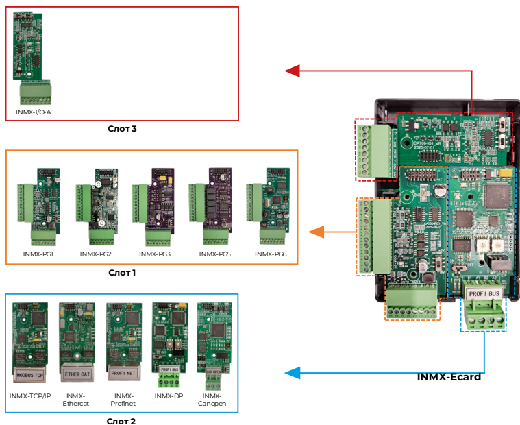
Рисунок 9.1 – Установка плат в модуль INMX-Ecard
