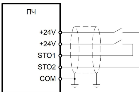
Рисунок 9.3 – Схема подключения для работы функции STO
