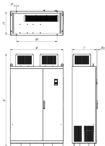
Рисунок 2.7 – Габаритные и установочные размеры устройств серии INPRIME MX в металлическом корпусе (напольное исполнение), типоразмеры 14-16
