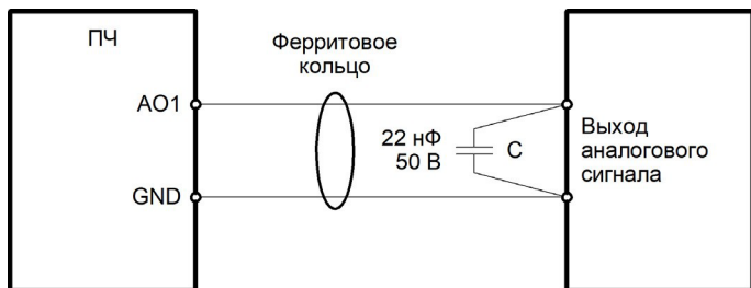
Рисунок 3.20 - Схема подключения проводов к аналоговому выходу (при воздействии сильных помех)
