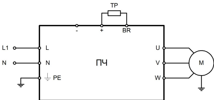
Рисунок 3.3 – Схема силовых подключений для моделей INPRIME MX-GY-2B
