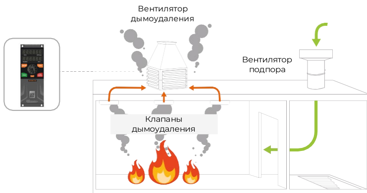
Рисунок 9.6 – Иллюстрация работы пожарного режима
