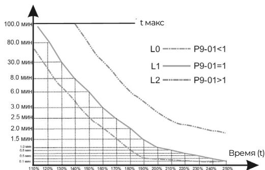
Рисунок 6.18 – Обратнозависимая времятоковая характеристика
