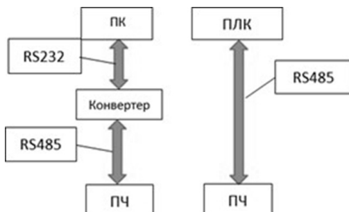
Рис. 7.1 Сетевой режим Master/Slave
