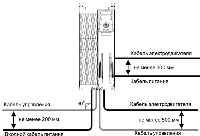
Рисунок 3.11 – Графическое представление расстояний между кабелями
