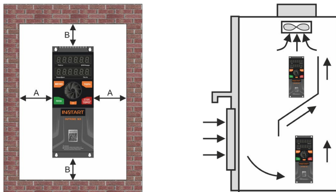
Рисунок 3.1 – Схема установки ПЧ серии INPRIME MX
