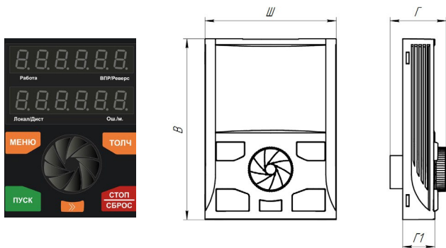
Рисунок 5.2 – Выносная панель управления INPMX-KP-LED
