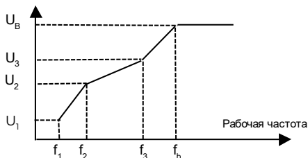
Рисунок 6.7 – Ломаная характеристика U/f
