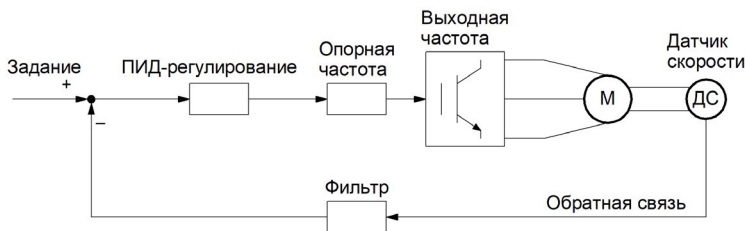
Рисунок 6.20 – Схема ПИД-регулирования
