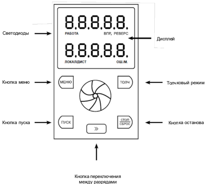
Рисунок 5.1 – Функции кнопок и светодиодов панели управления INPRIME MX
