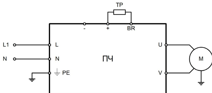
Рисунок 3.2 – Схема силовых подключений для моделей INPRIME MX-GY-1B
