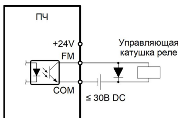
Рисунок 3.19 – Подключение к цифровому выходу с использованием внешнего источника питания
