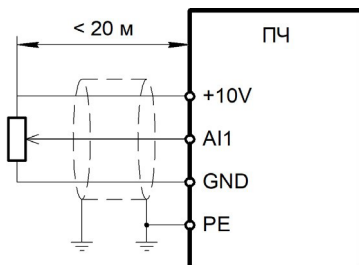
Рисунок 3.13 – Схема подключения проводов к аналоговому входу (общий случай)
