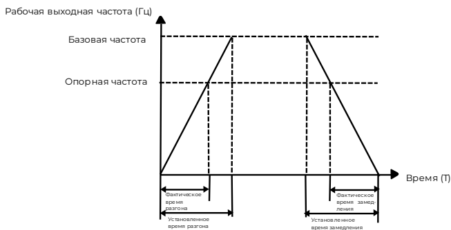
Рисунок 6.3 – Время разгона/замедления
