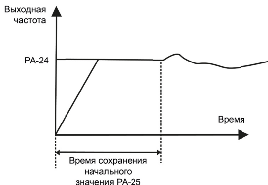
Рисунок 6.22 – Время сохранения опорного значения
