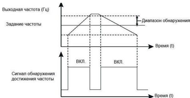
Рисунок 6.17 – Диапазон достижения максимальной частоты
