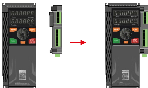
Рисунок 5.5 – Установка модуля INMX-Ecard в моделях до 22 кВт (включительно)
