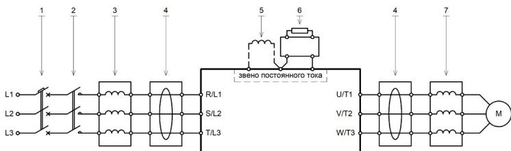
Рисунок 3.6 – Схема подключения дополнительного оборудования
