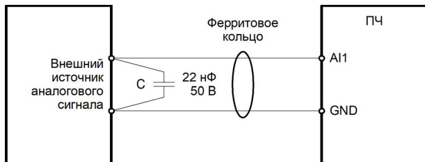
Рисунок 3.14 – Схема подключения проводов к аналоговому входу (при воздействии сильных помех)
