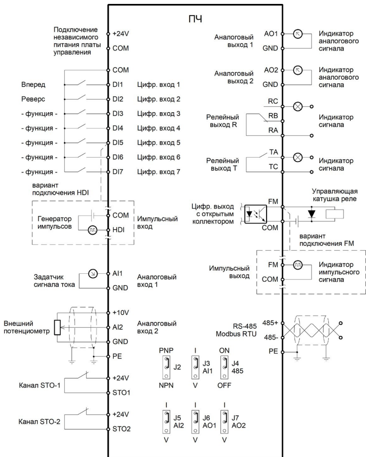
Рисунок 3.8 – Схема подключения управляющих клемм серии INPRIME MX
