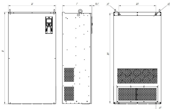
Рисунок 2.6 – Габаритные и установочные размеры устройств серии INPRIME MX в металлическом корпусе (настенное исполнение), типоразмеры 5-13
