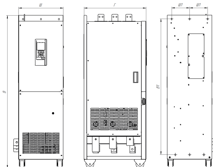
Типоразмеры 9-10 серии INPRIME
