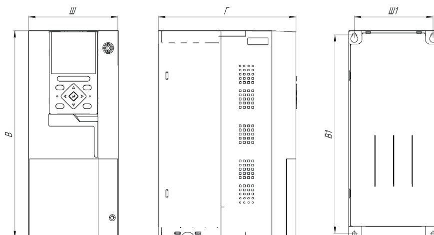
Типоразмеры 1-8 серии INPRIME
