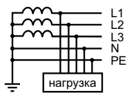
Схема TN-S
