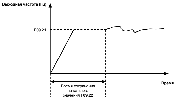
Рисунок 6.18 – Время сохранения опорного значения
