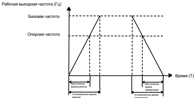
Рисунок 6.2 – Время разгона/замедления
