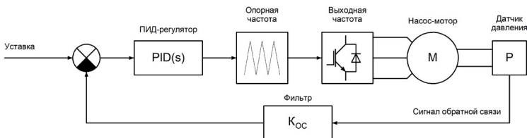
Рисунок 6.16 – Схема ПИД-регулирования
