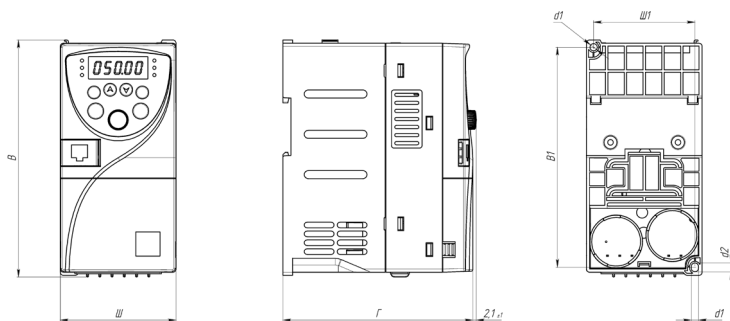
Рисунок 2.4 – Габаритные и установочные размеры устройств серии INVENT типоразмера 1
