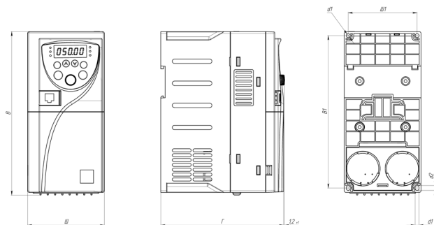
Рисунок 2.5 – Габаритные и установочные размеры устройств серии INVENT типоразмера 2
