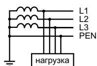
Схема TN-C
