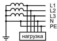
Схема TN-C-S
