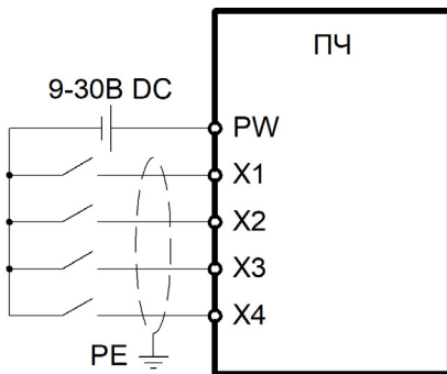
Рисунок 3.16 – Схема подключения, при которой используется внешний источник питания, цифровые входы в режиме NPN
