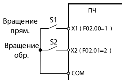
Рис.7.2а Двухпроводное управление F00.03=1
