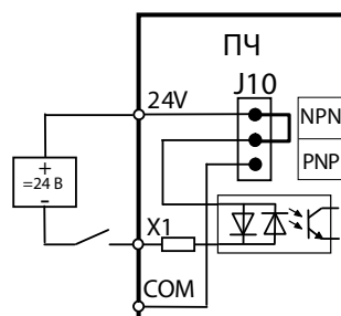
Логика PNP от внутреннего источника питания «+24V». Перемычка J10 в положении PNP
