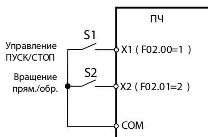
Рис.7.1а Двухпроводное управление F00.03=0
