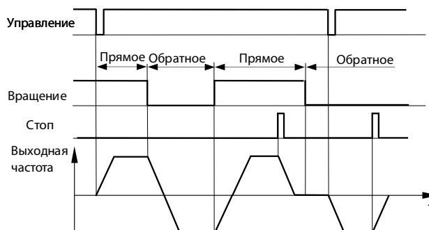
Рис.7.4б Двухпроводное управление F00.03=3, F04.19=0
