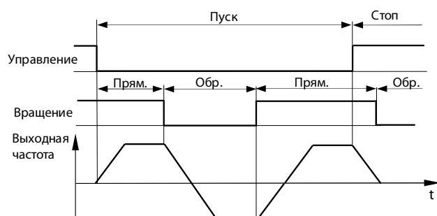
Рис.7.1б Двухпроводное управление F00.03=0, F04.19=0
