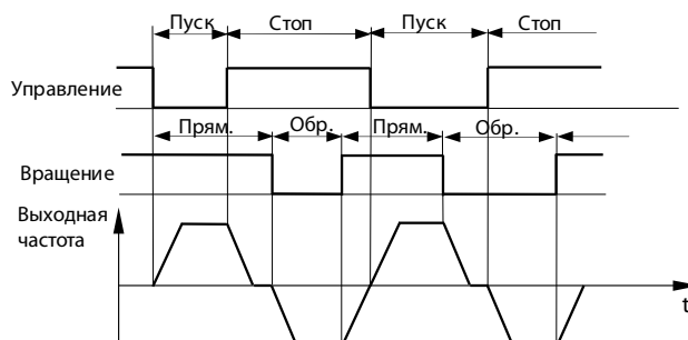
Рис.7.2б Двухпроводное управление F00.03=1, F04.19=0
