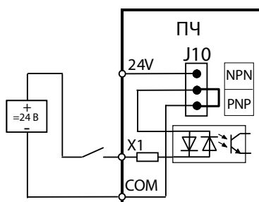
Логика NPN от внешнего источника питания 24 В. Перемычка J10 в положении NPN.
