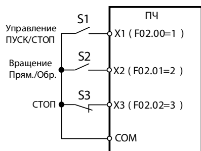
Рис.7.4а Двухпроводное управление F00.03=3
