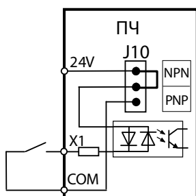
Логика NPN от внутреннего источника питания «+24V». Перемычка J10 в положении NPN.
