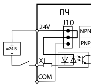
Логика PNP от внешнего источника питания 24 В. Перемычка J10 в положении PNP.
