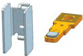
Конструкция, предотвращающая плавление контактов
