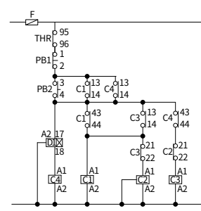
Схема подключения 2 (HGC115 ~ 800)
