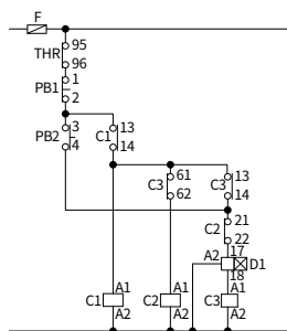
Схема подключения 1 (HGC9 ~ 100)
