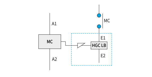
Электрическая схема
