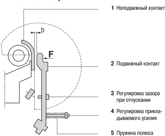
Регулировка НЗ полюса автоматического отключения катушки
