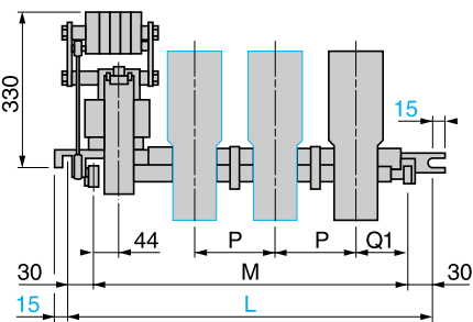
Контакты CV3 и LC1 В: 1-полюсные, 2-полюсные или 3-полюсные
