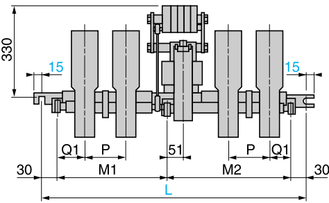
Контакты CV3 и LC1 В, 4-полюсные
