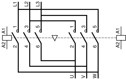
Реверсивные контакты для управления электродвигателями, горизонтального крепления LC2-F 2 x LC1-F
