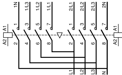
Контакты автоматического ввода резерва для распределительных сетей, горизонтального крепления LC2-F 2 x LC1-F
