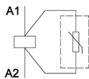
Варистор
