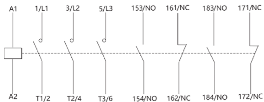
MC1G 3P
