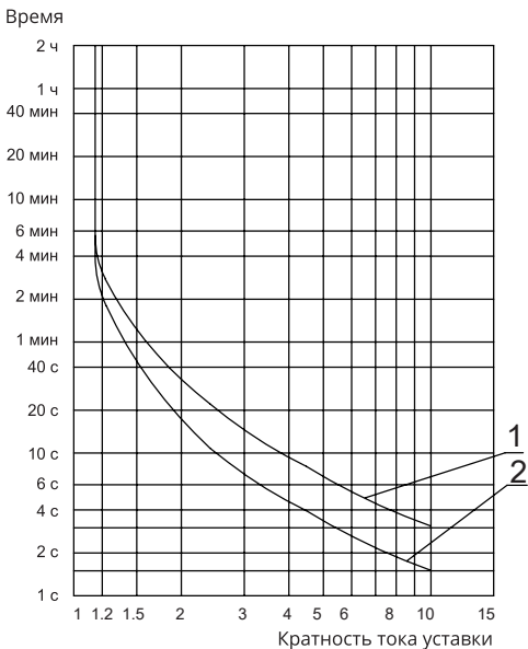
Характеристика срабатывания при обрыве одной фазы
