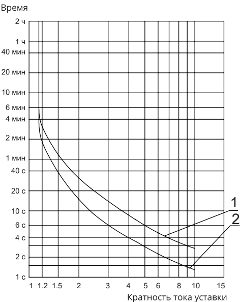
Характеристика срабатывания при симметричной трехфазной нагрузке
