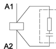
R-С цепочка
