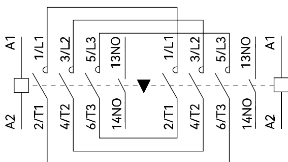
MC2Kxx10xx
