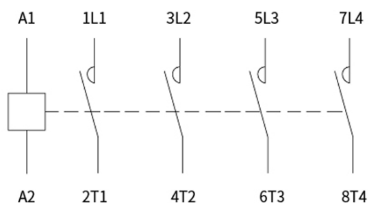
MC(P)1K08xx
