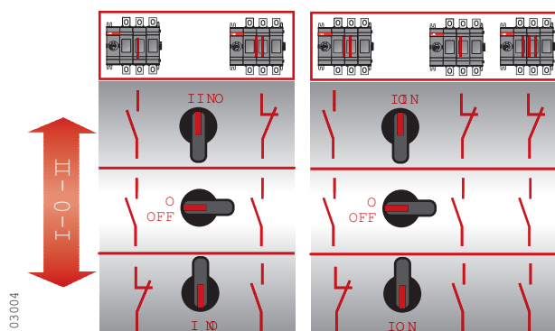
Принцип работы реверсивной блокировки
