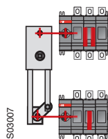
Реверсивная блокировка
