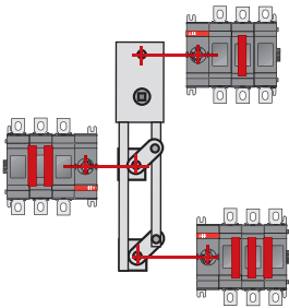
Байпасная блокировка
