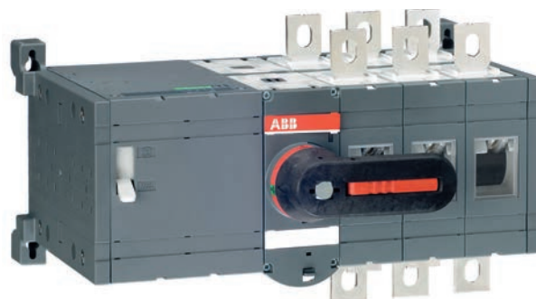
Реверсивный рубильник с моторным приводом OTM250E3CM230C на базе ОТ
