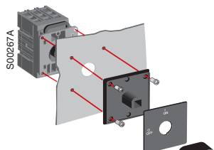
Крепление на винтах
