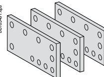
Контактные пластины для присоединения кабелей с наконечниками
