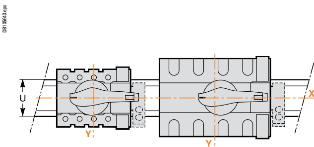
Размеры (мм)
