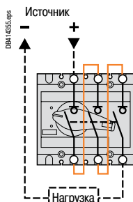
Последовательное соединение полюсов на вводе / отходящих линиях (осуществляется заказчиком)
