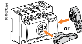
Стандартная поворотная рукоятка: INS40 - 160
