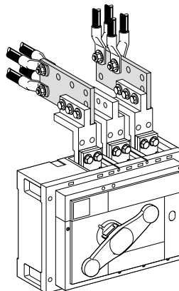
Расширители полюсов
