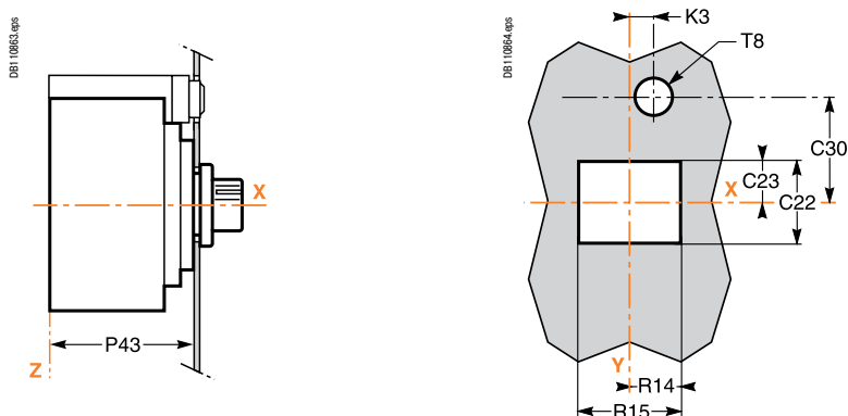
Размеры (мм)
