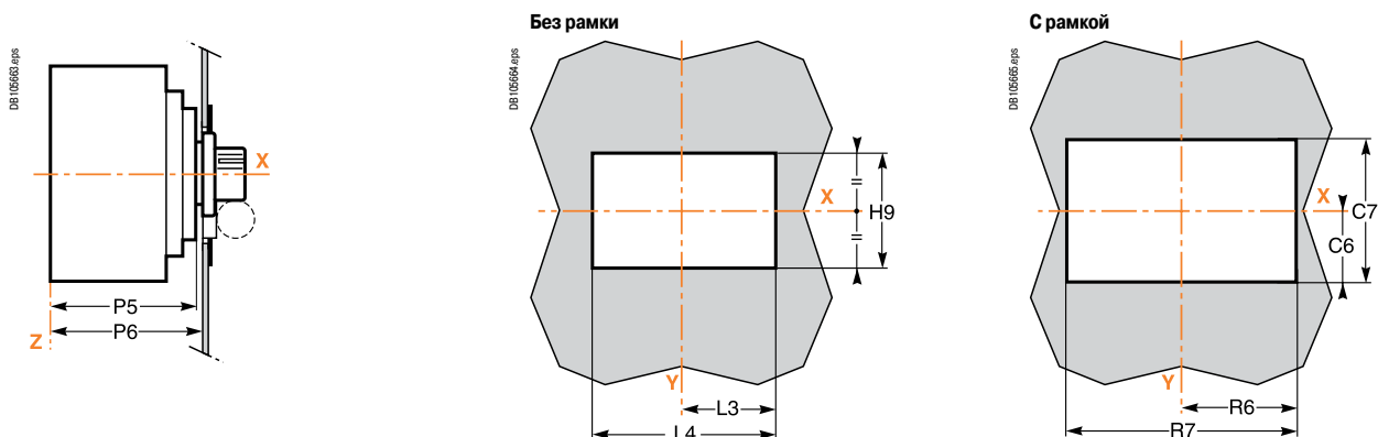
Размеры (мм)
