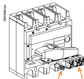
Compact INS/INV320 - 630
